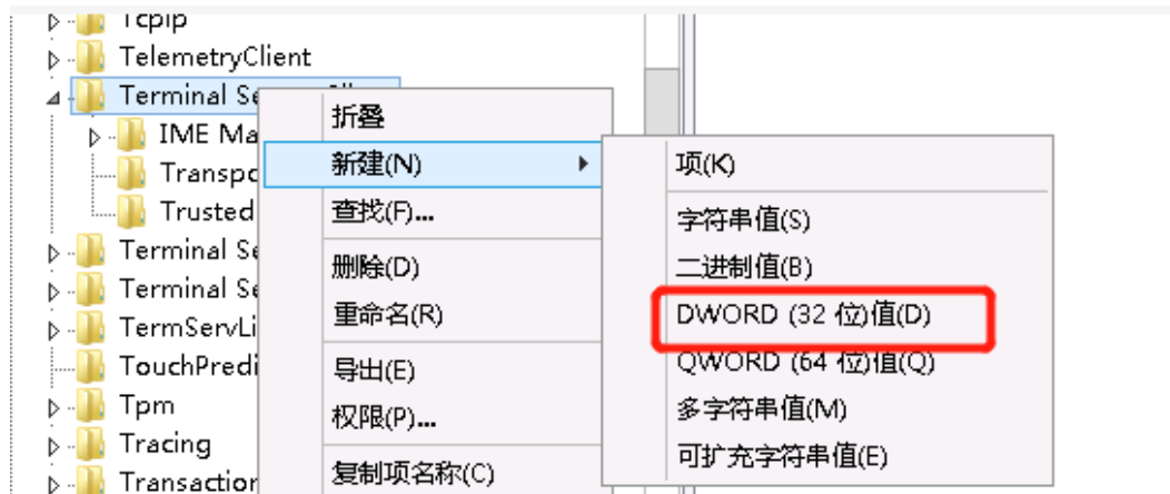
图 13-7 新建 DWORD
