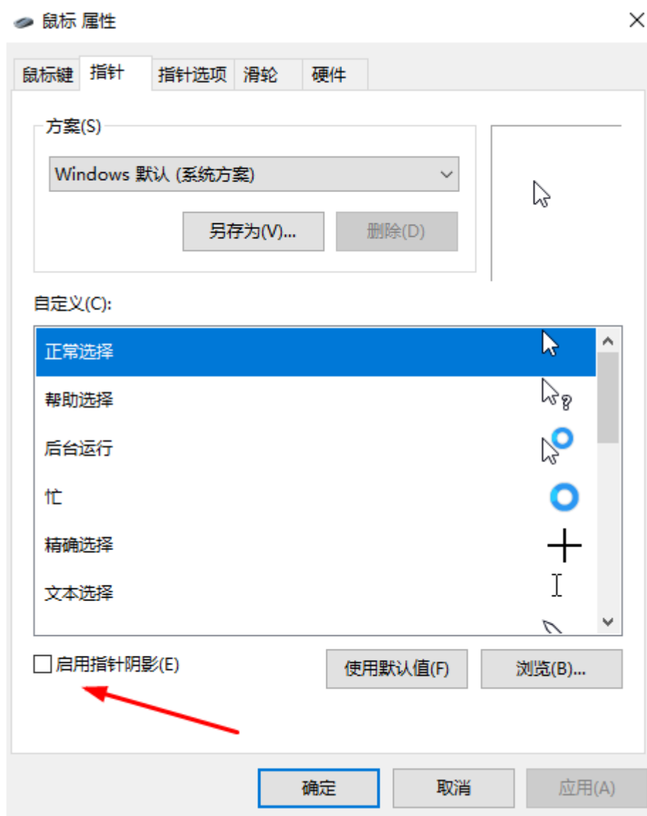
图 13-14 指针
