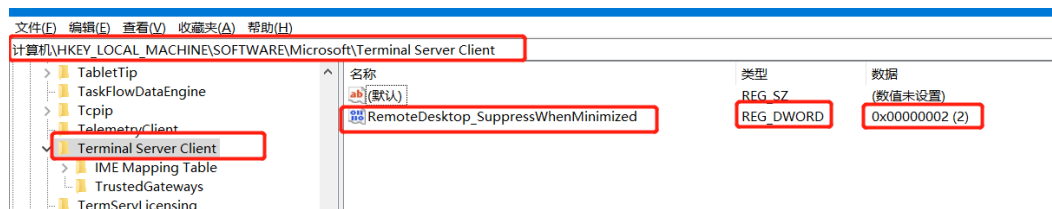
图 13-8 设置值大小
