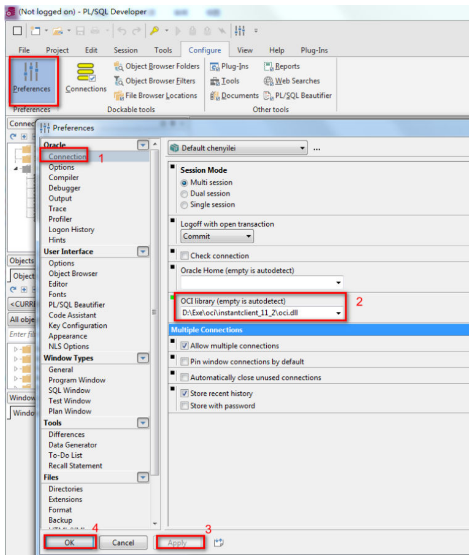
图 13-15 配置文件
