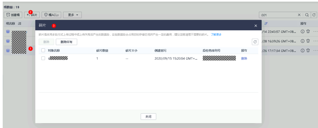
图 6-5 碎片管理
