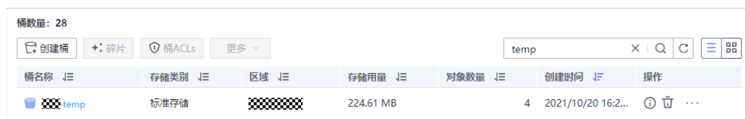
图 6-3 搜索桶
