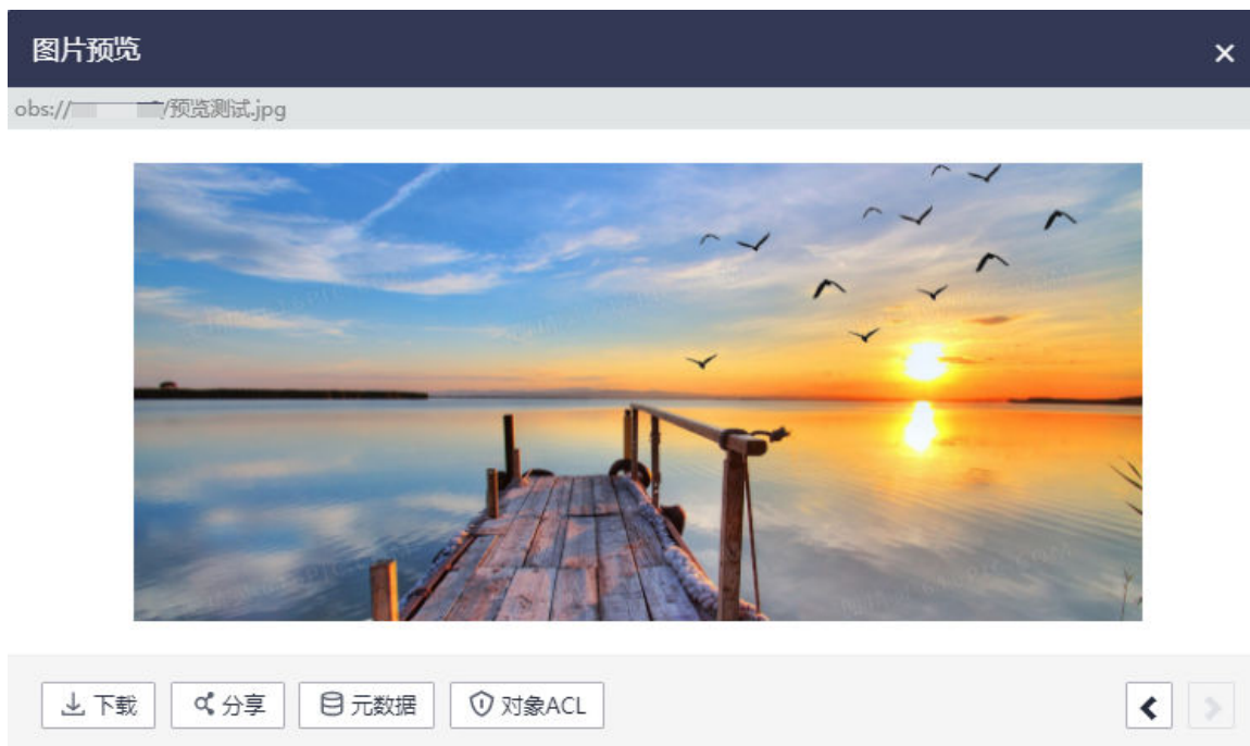
图 8-12 预览对象
