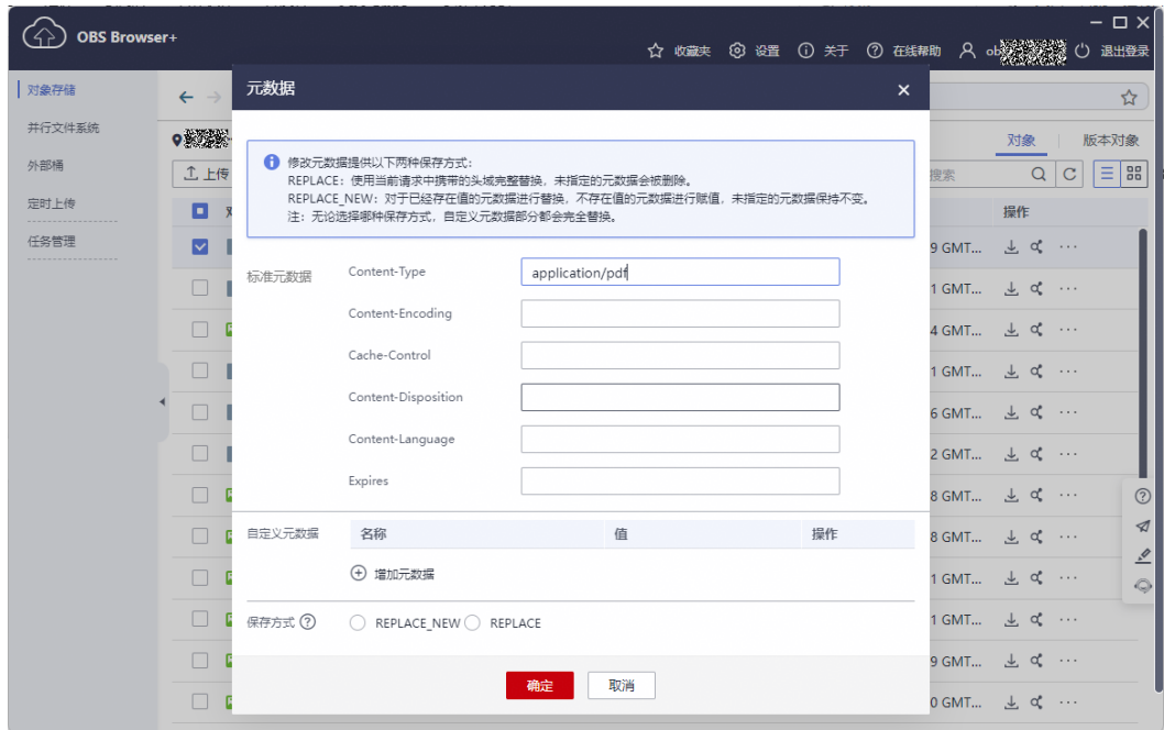
图 8-5 对象元数据
