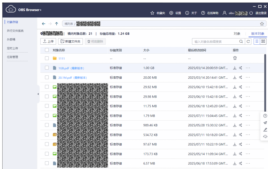
图 8-3 版本对象
