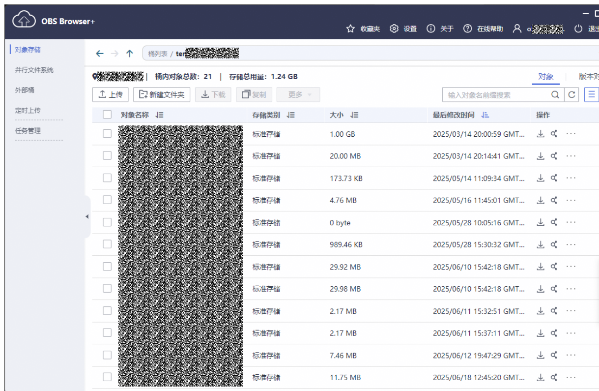
图 8-2 对象列表
