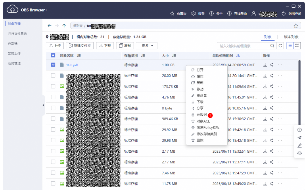
图 8-4 对象管理
