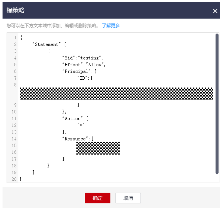
图 7-4 桶策略
