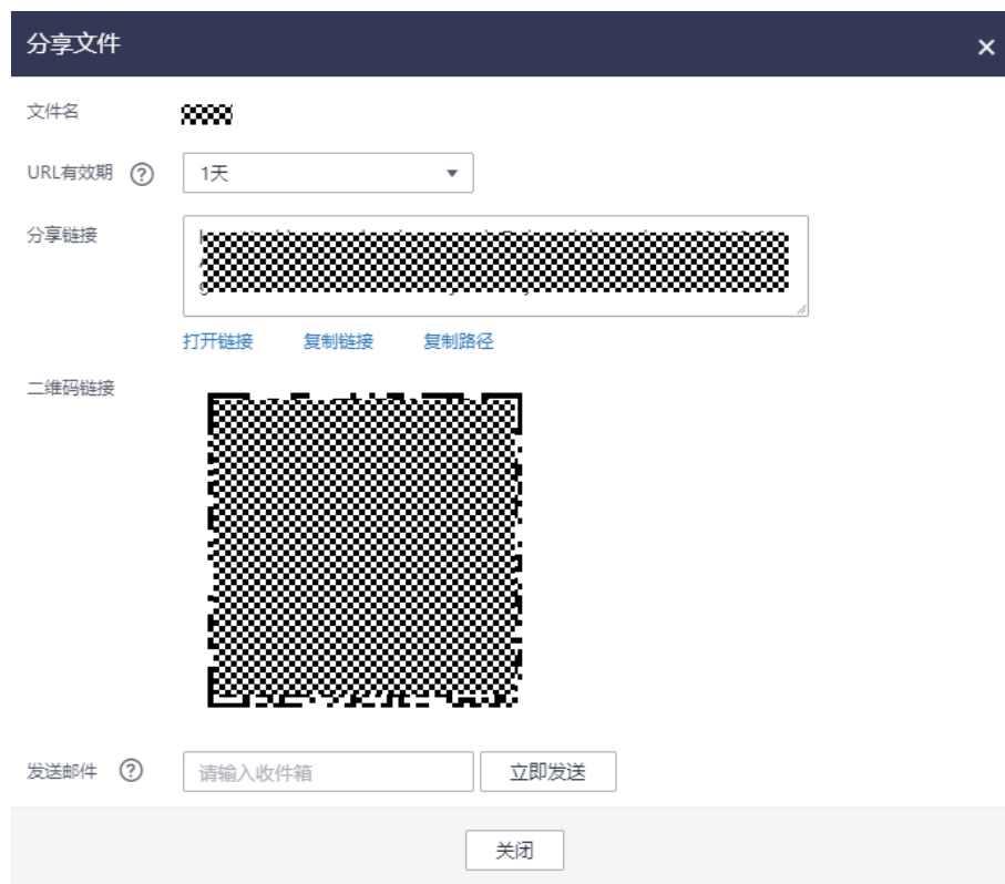
图 8-9 分享文件
