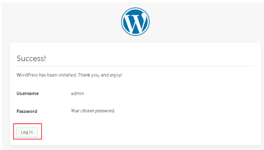
图 3-27 安装成功
