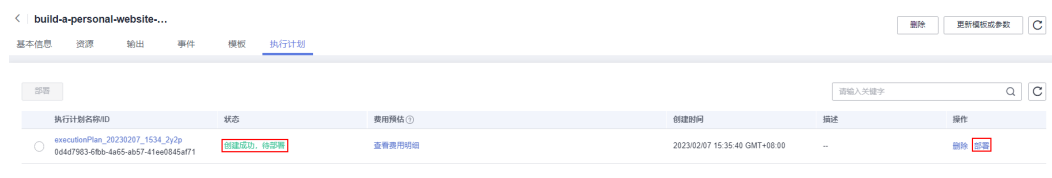
图 3-14 执行计划
