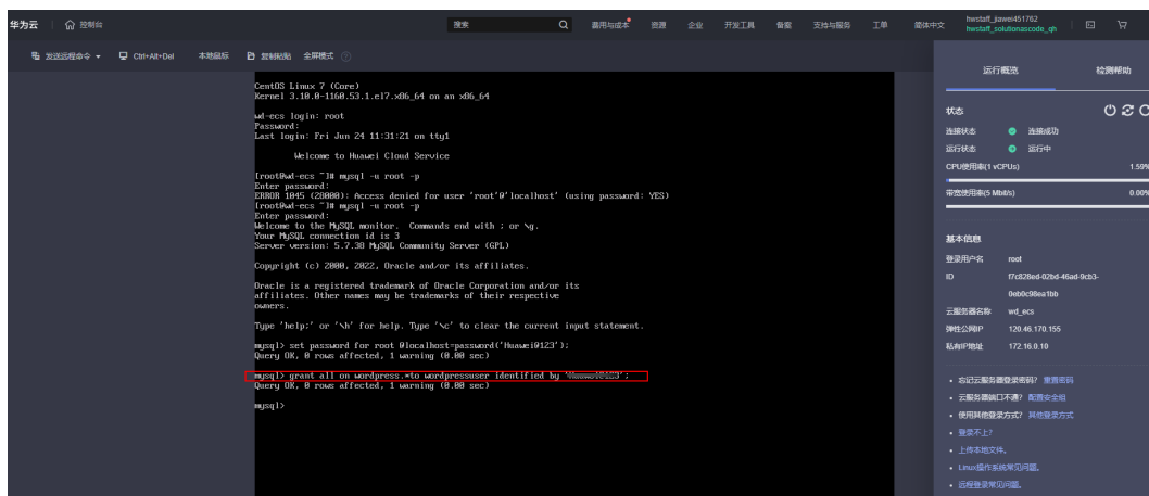
图 3-21 修改 MySQL 数据库的 database 用户密码
