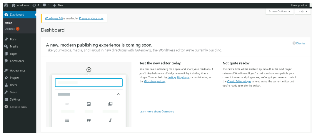
图 3-29 WordPress 界面
