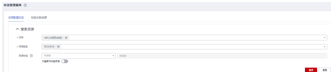
图 2-1 搜索资源
