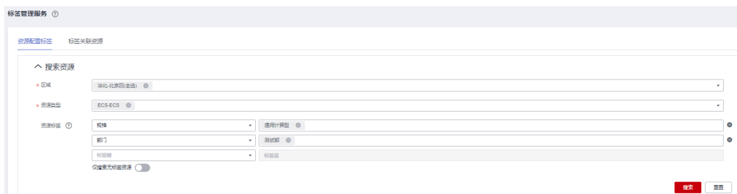
图 2-3 搜索资源
