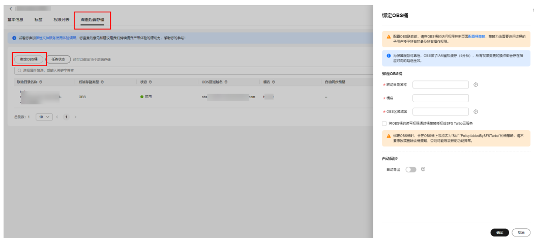
图 4-5 绑定 OBS 桶
