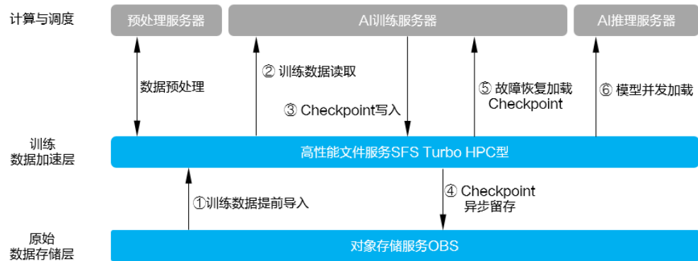
图 6-1 基于 OBS+SFS Turbo 的华为云 AI 云存储解决方案
