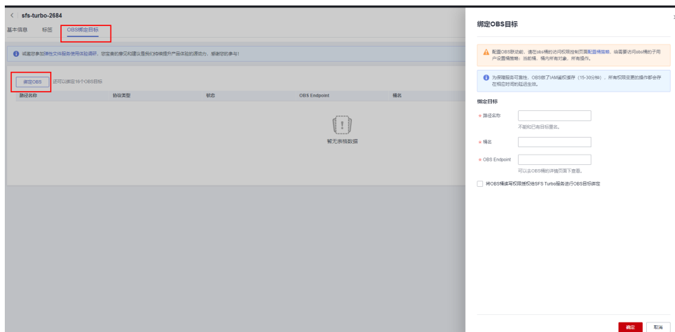
图 6-5 绑定 OBS 桶
