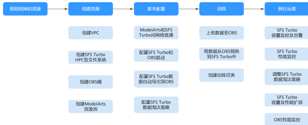
图 6-2 面向 AI 场景使用 OBS+SFS Turbo 的存储加速方案步骤
