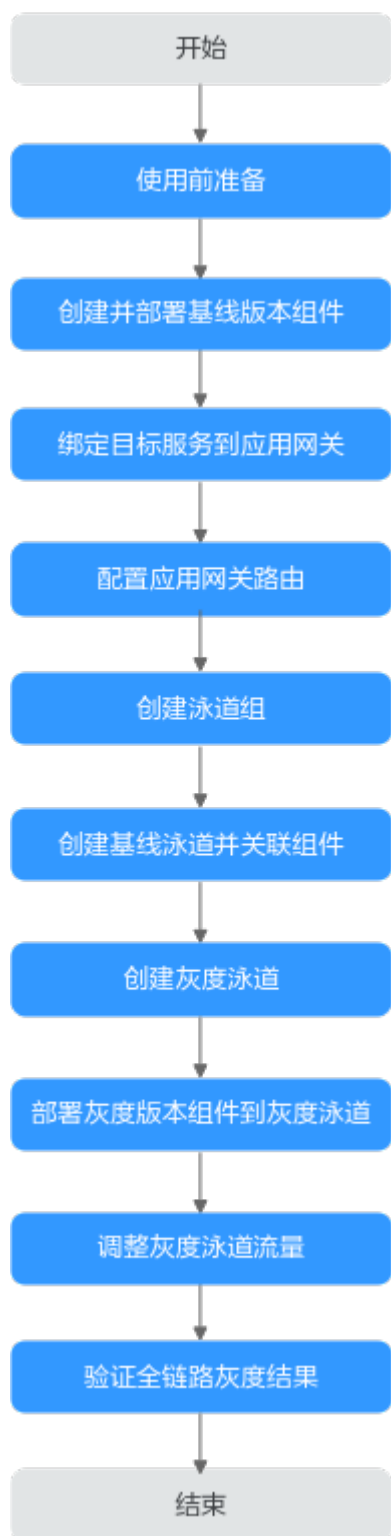
图 8-2 全链路流量控制使用流程
