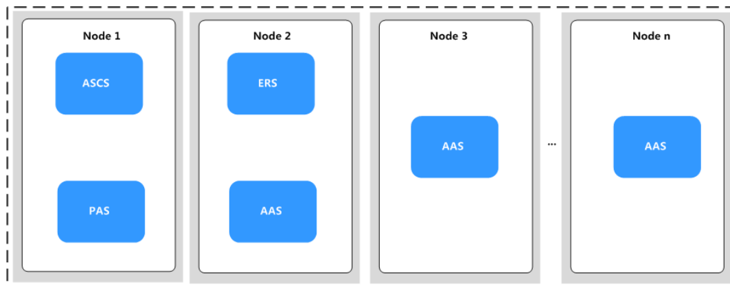
图 6-4 SAP S/4HANA (HA+分布式) 部署方案
