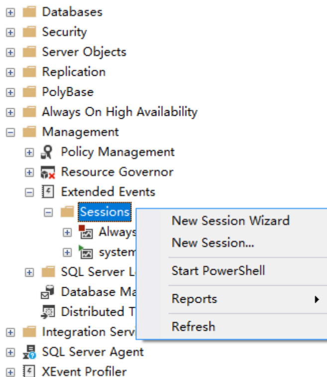
图 4-67 新建事件
