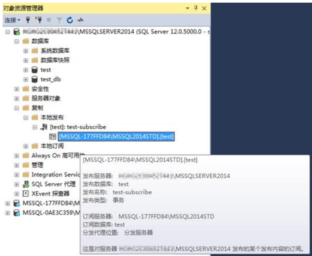
图 4-39 查看订阅
