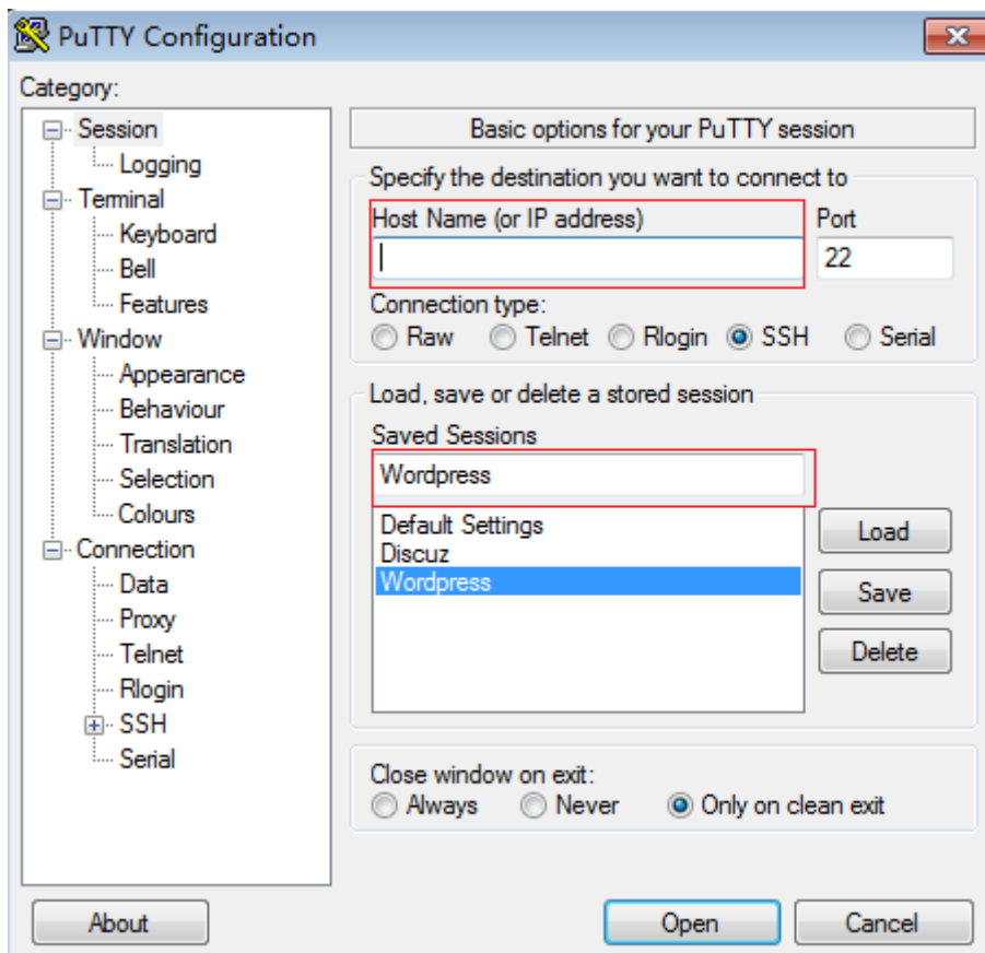
图 2-46 配置 PuTTY
