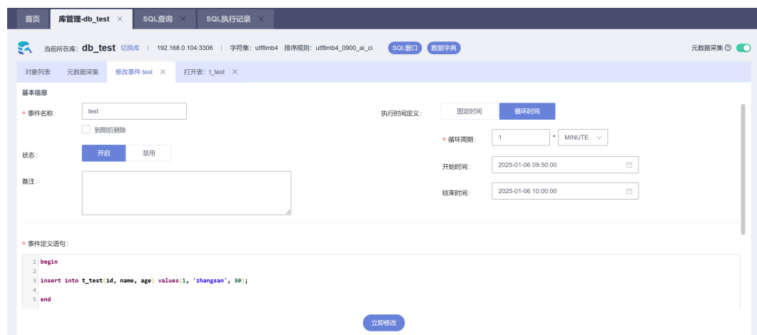
图 2-67 新建事件
