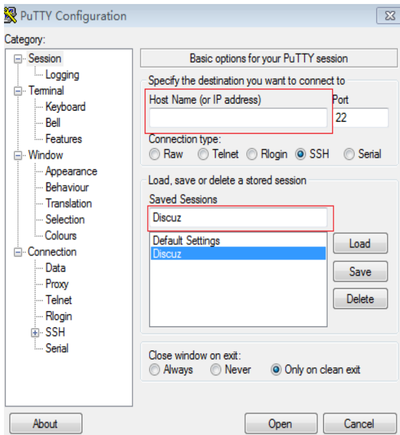
图 2-57 配置 PuTTY
