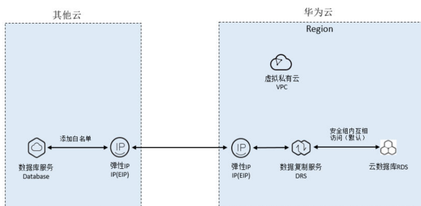
图 2-33 部署架构图
