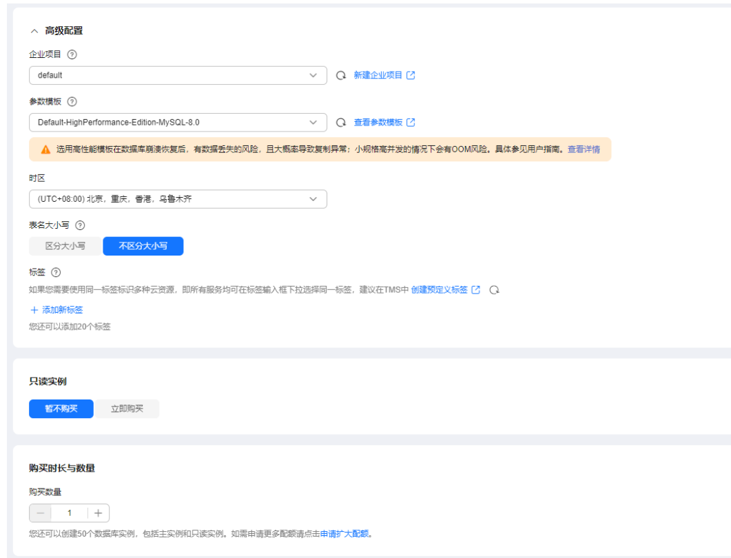
图 2-16 高级配置
