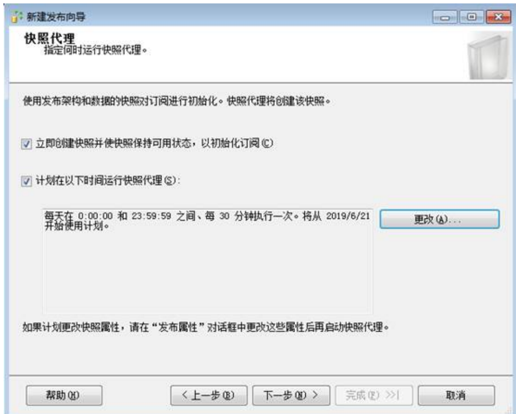
图 4-27 快照代理
