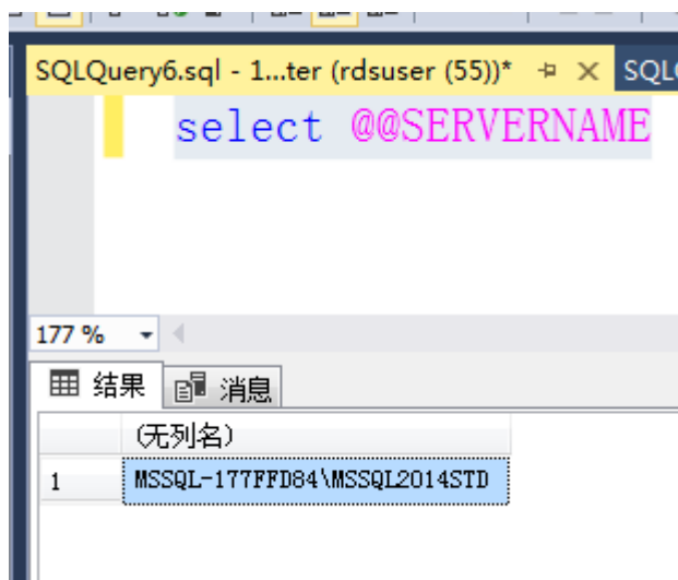
图 4-21 设置别名
