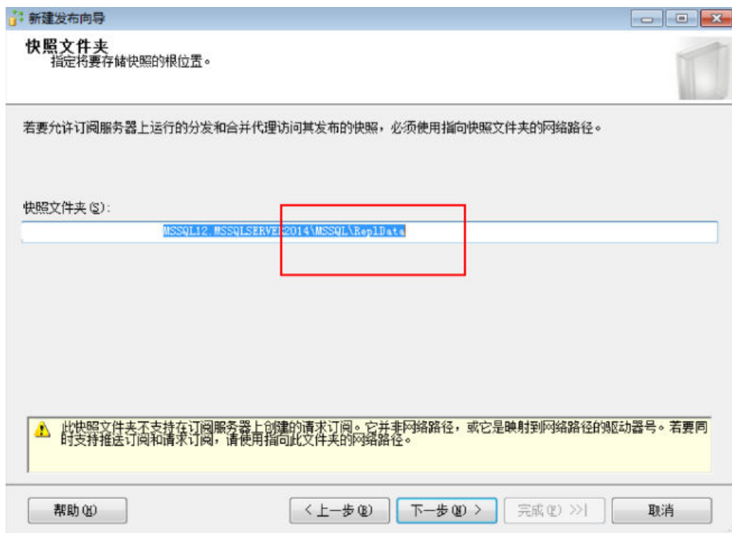
图 4-16 快照文件夹
