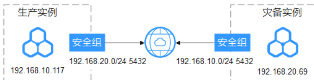
图 3-18 防火墙配置
