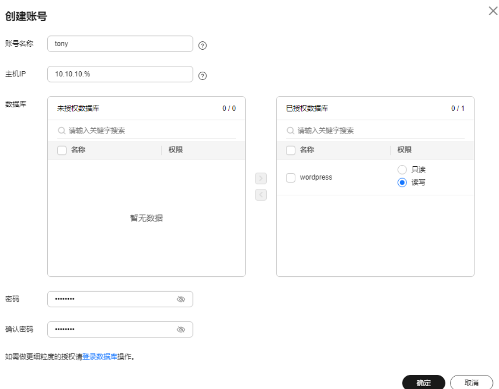
图 2-48 创建账号
