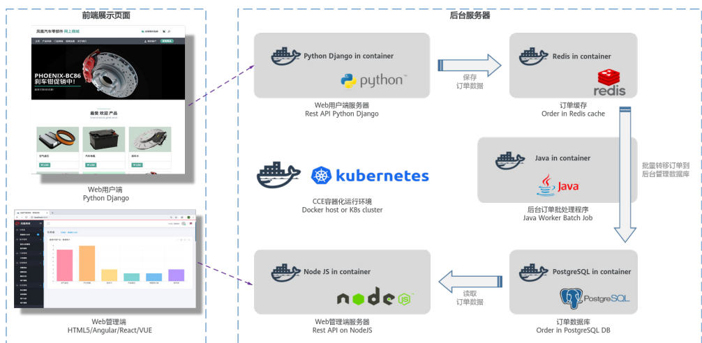
图 8-2 凤凰商城技术架构图
