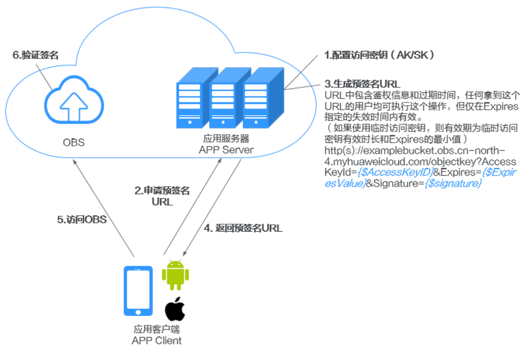
图 2-4 移动应用访问 OBS 数据流程
