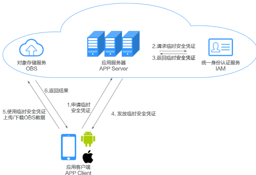
图 15-1 使用临时安全凭证直传 OBS 流程
