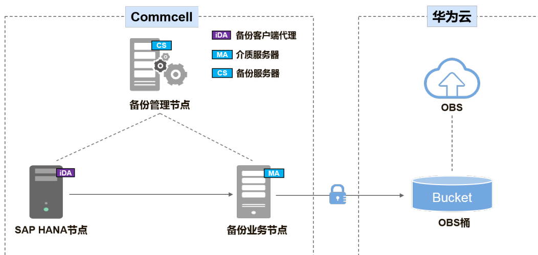
图 7-1 逻辑架构
