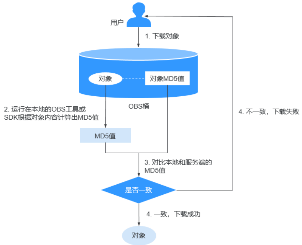
图 11-2 校验下载对象的一致性
