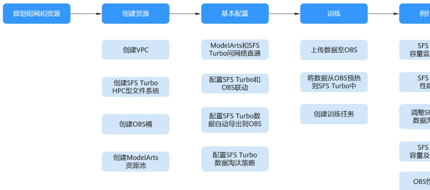
图 19-2 面向 AI 场景使用 OBS+SFS Turbo 的存储加速方案步骤
