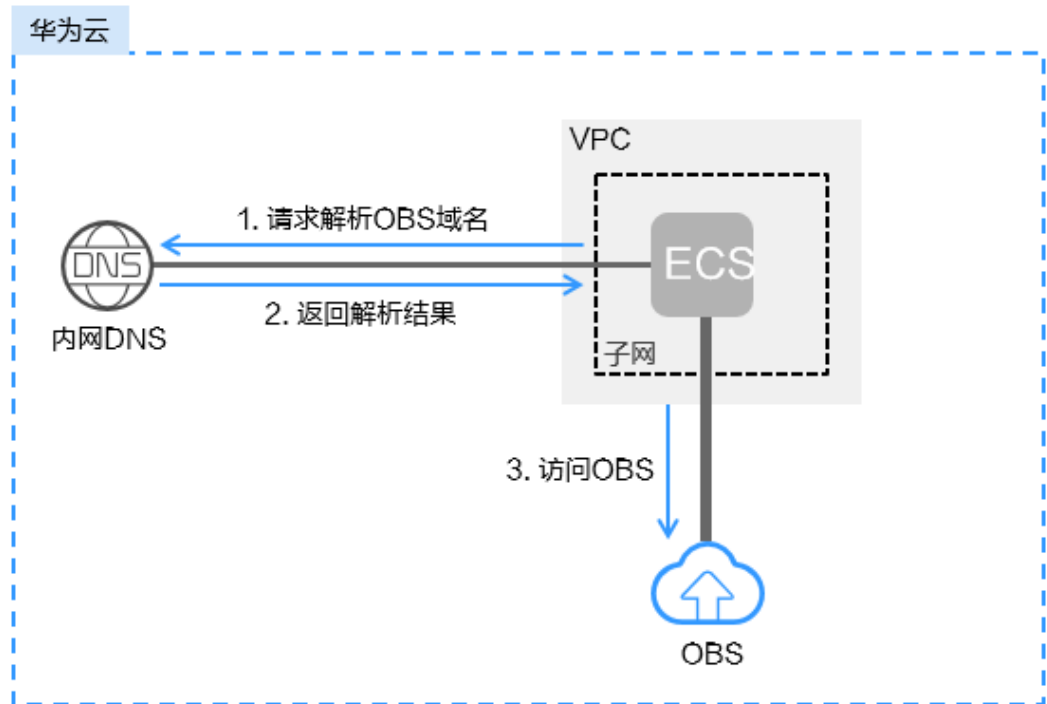
图 8-1 内网访问 OBS 示意图
