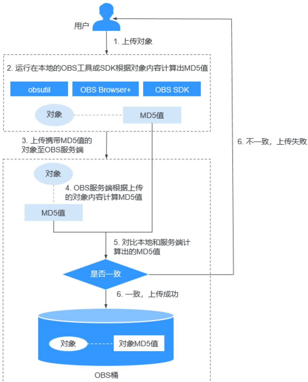
图 11-1 校验上传对象的一致性
