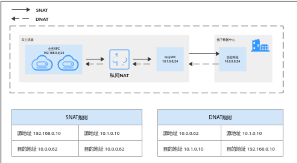
图 4-1 组网图
