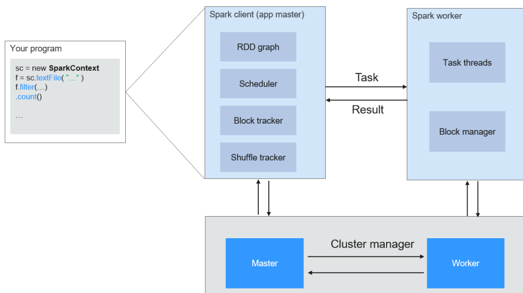
图 2-1 Spark 应用运行架构
