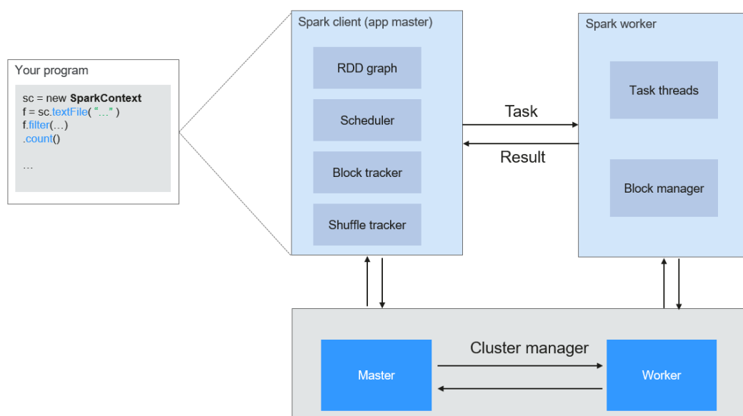
图 4-5 Spark 应用运行架构
