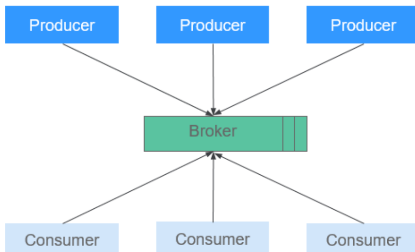
图 5-37 Kafka 结构
