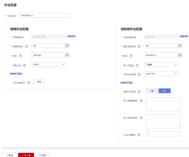
图 2-39 新建作业
