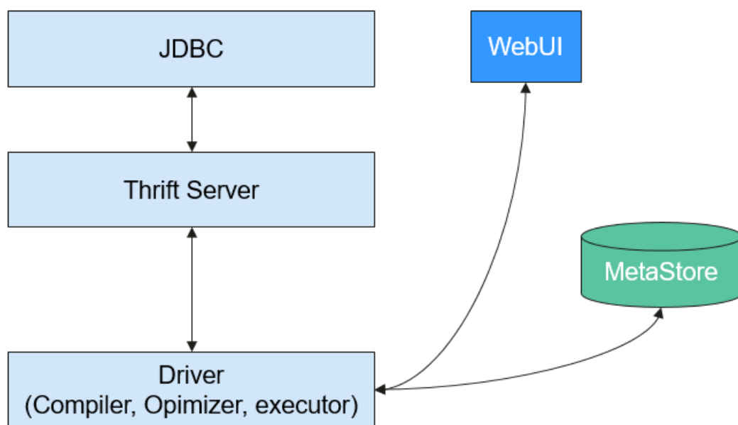
图 4-14 Hive 结构
