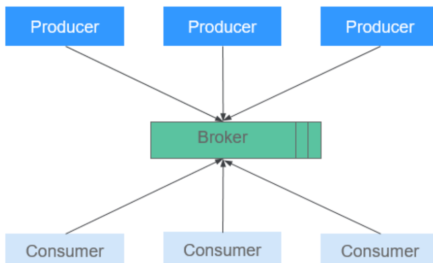
图 2-28 Kafka 结构
