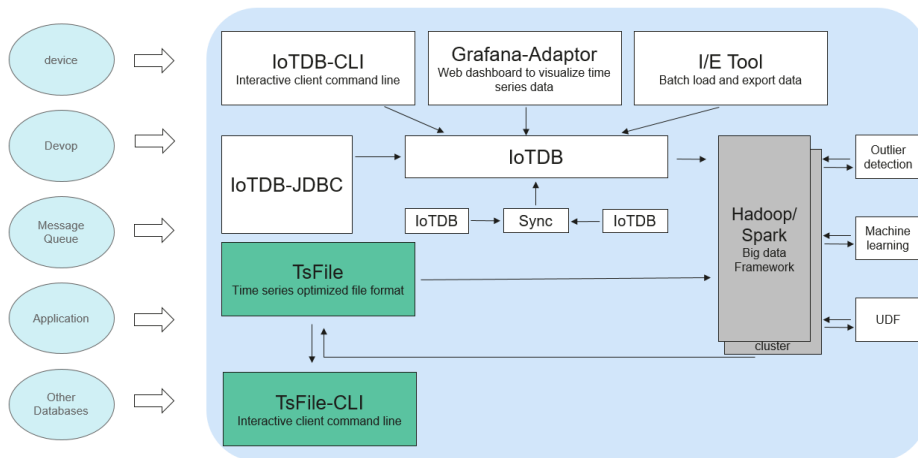
图 2-60 IoTDB 结构
