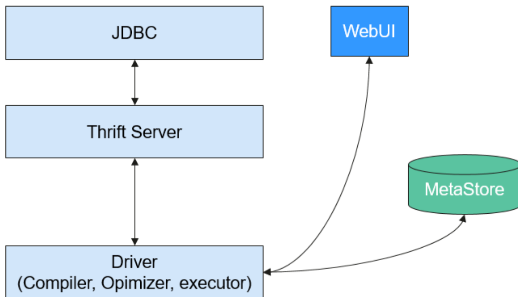
图 2-10 Hive 结构
