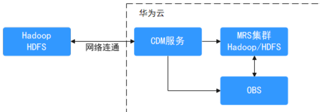
图 3-7 Hadoop 数据迁移示意
