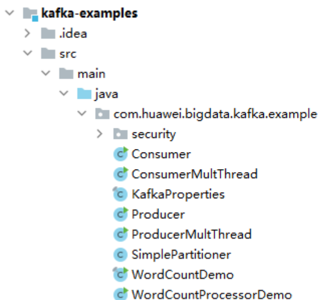
图 2-29 导入 Kafka 样例程序
