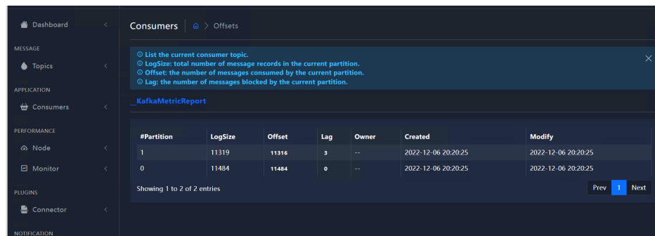
图 5-41 Consumer 监控
