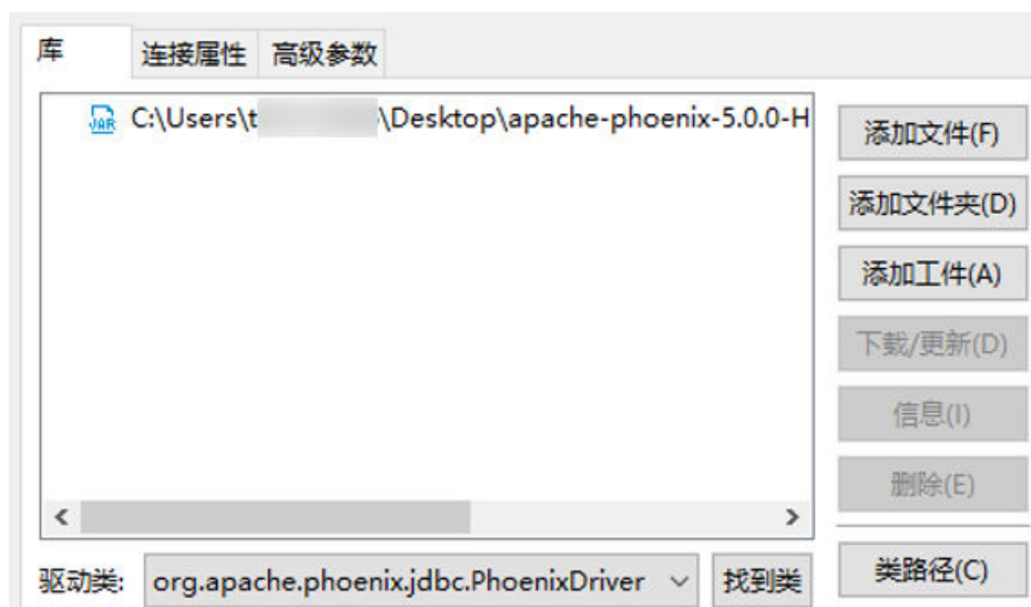
图 5-8 加载驱动类
