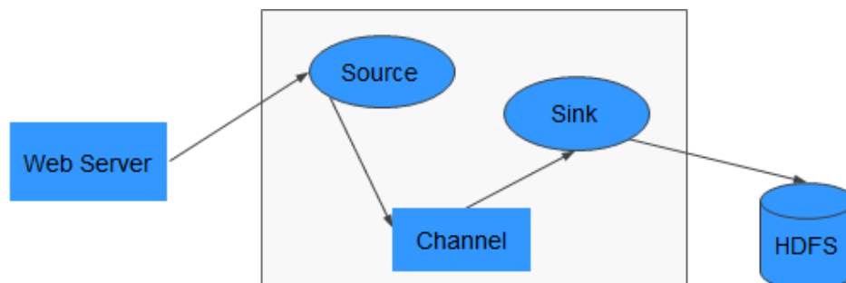
图 2-20 Flume-NG 架构
