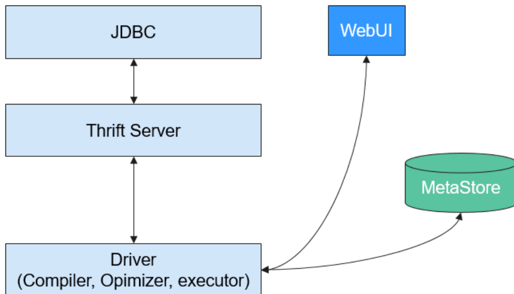
图 4-7 Hive 结构
