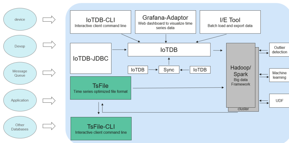
图 2-51 IoTDB 结构
