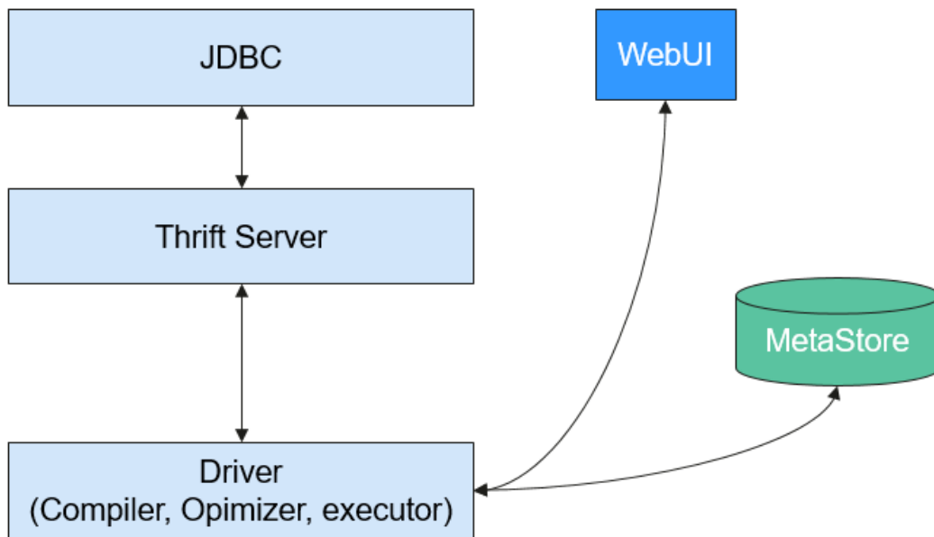
图 5-36 Hive 结构
