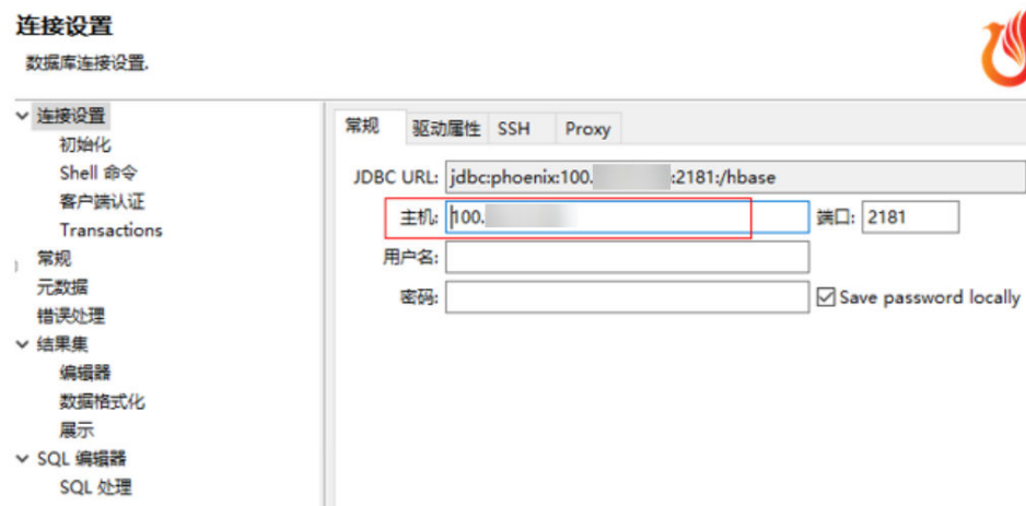
图 5-11 配置主机
