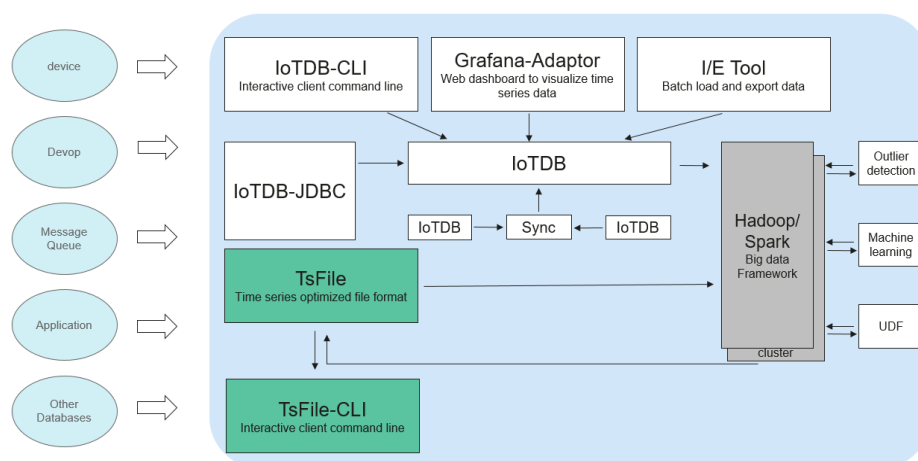
图 2-79 IoTDB 结构
