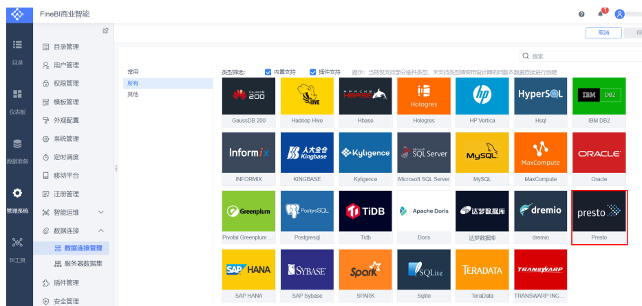
图 5-20 新建连接
