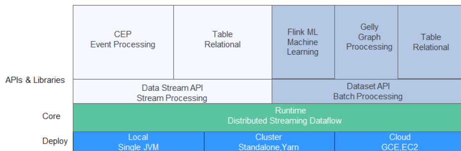
图 2-12 Flink 架构
