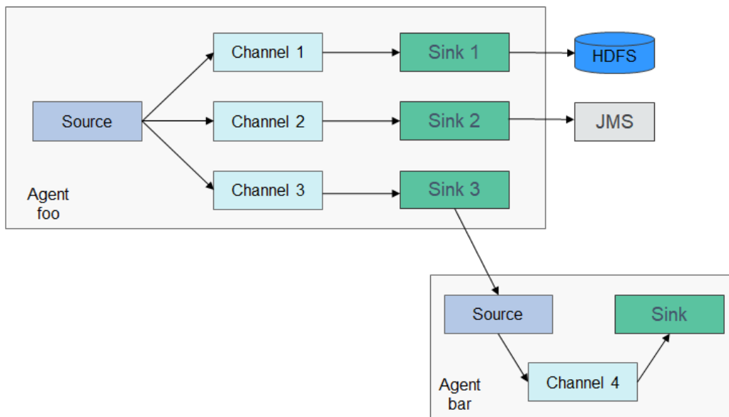
图 2-21 Flume 结构图
