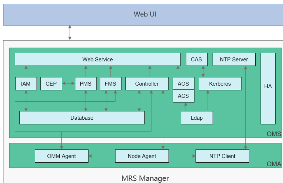
图 6-1 Manager 逻辑架构
