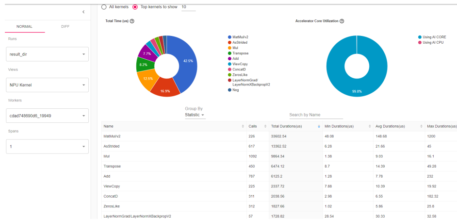
图 7-78 Kernel 视图
