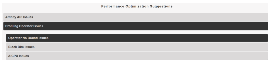
图 7-45 生成结果
