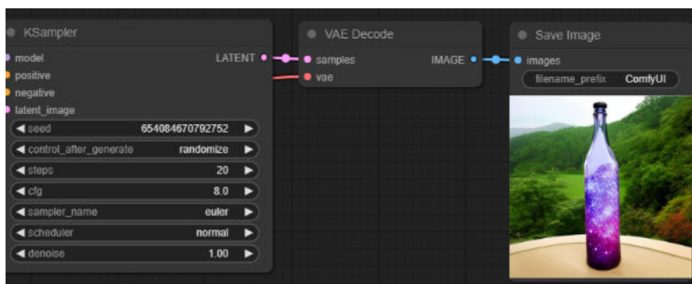
图 4-13 推理成功
