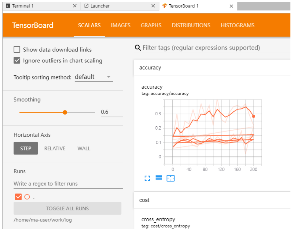
图 13-18 TensorBoard 界面 (3)
