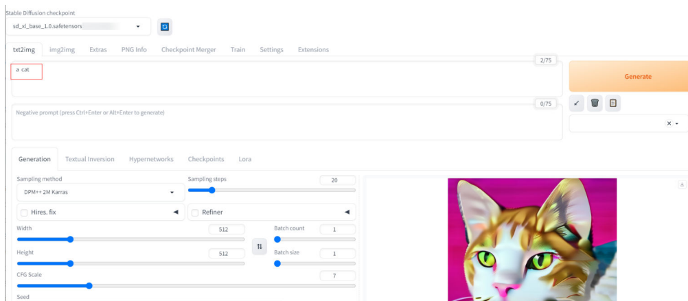
图 4-16 文生图
