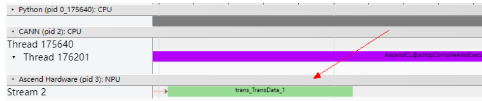
图 7-77 算子 TransData
