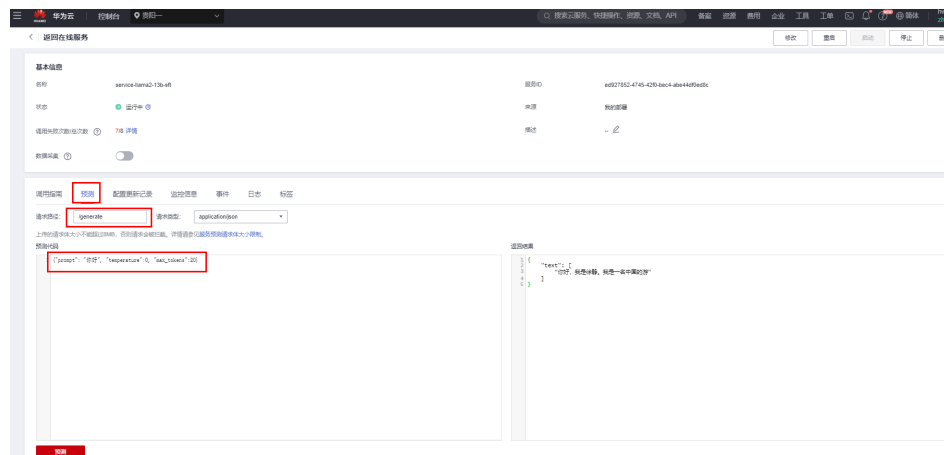
图 3-77 预测
