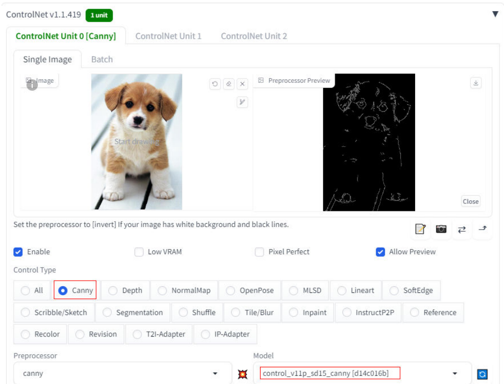
图 4-19 带 controlnet 运行
