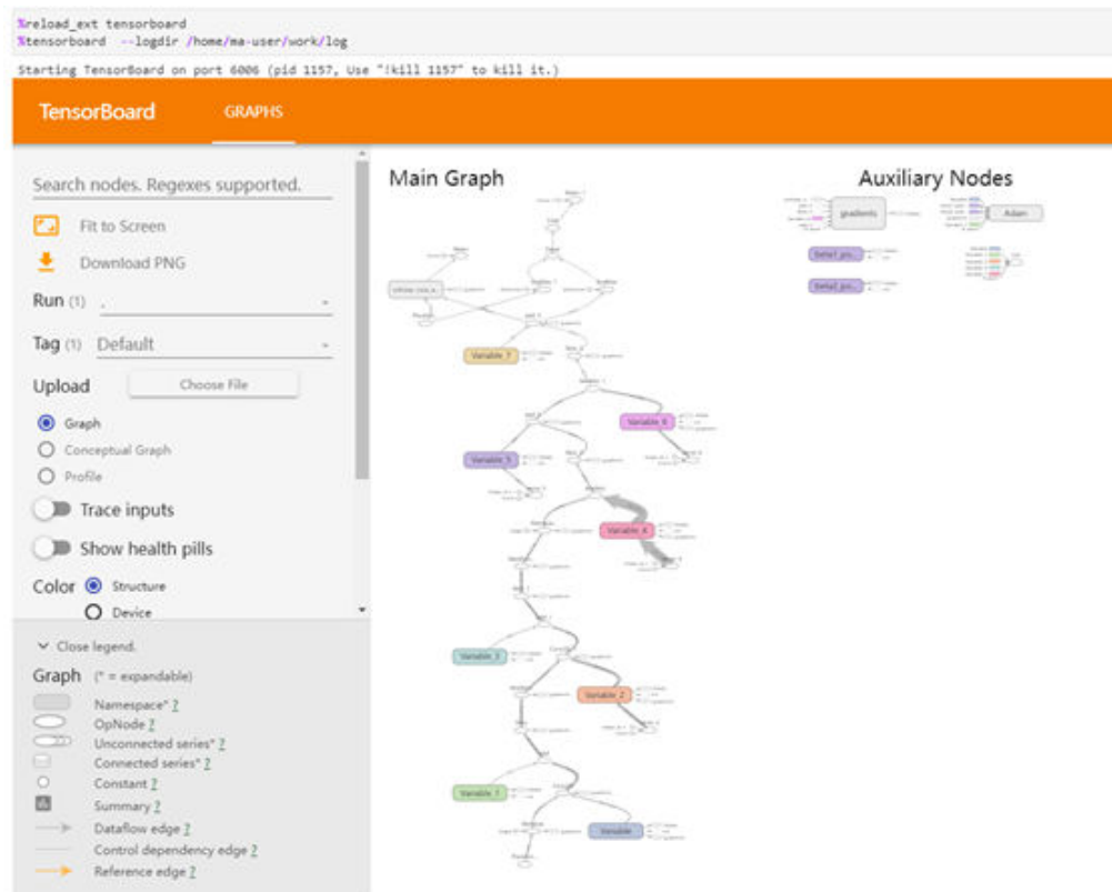
图 13-15 TensorBoard 界面 (2)
