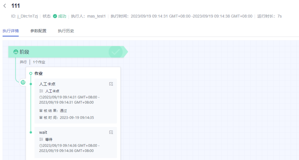
图 4-9 执行详情
