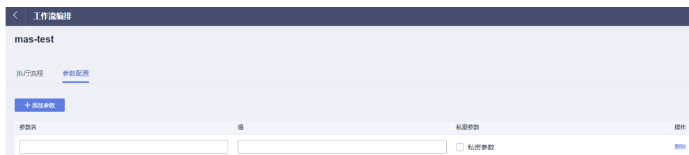
图 4-3 参数配置
