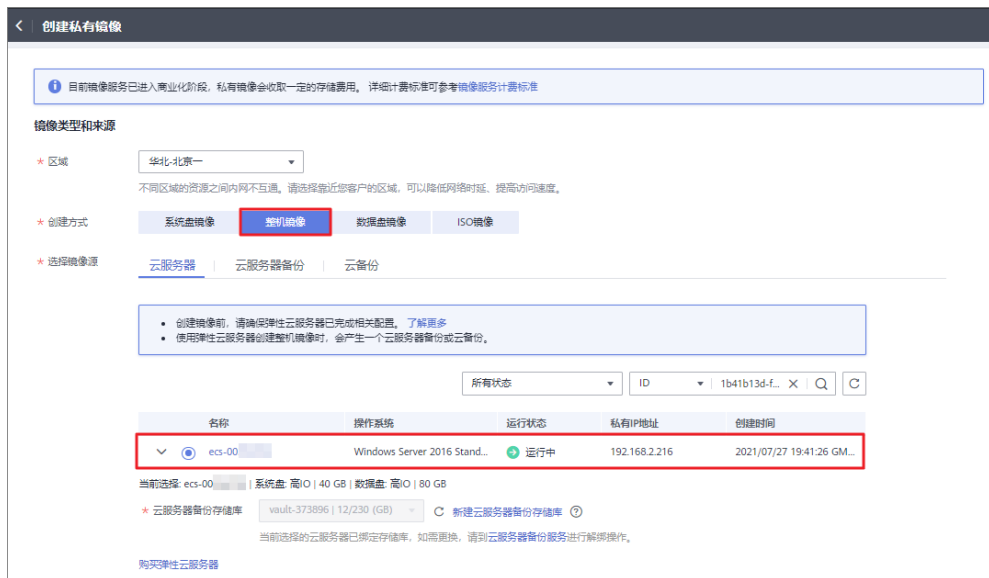
图 10-4 创建整机镜像
