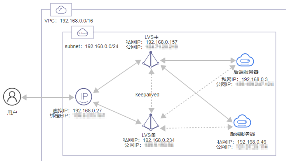
图 2-1 组网图
