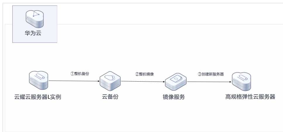
图 14-1 方案架构图
