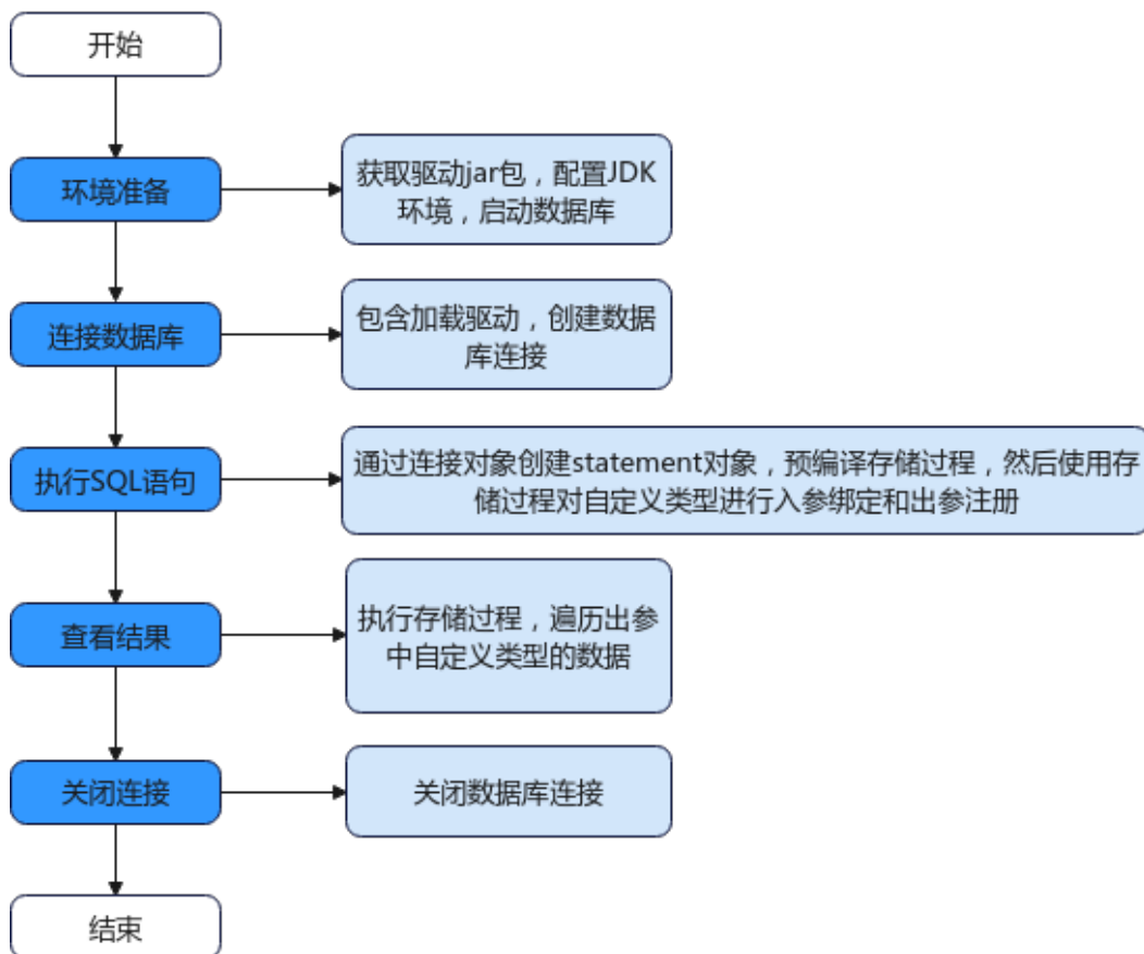
图 14-4 JDBC 使用存储过程操作自定义类型
