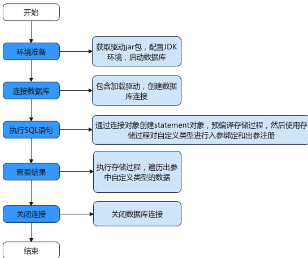
图 14-9 JDBC 使用存储过程操作自定义类型
