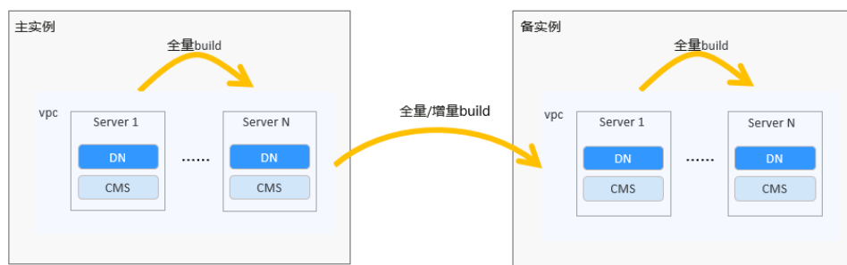
图 6-1 容灾原理图
