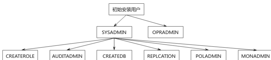
图 9-1 权限架构
