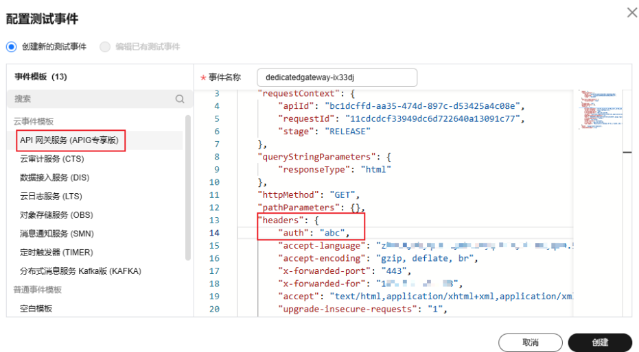
图 4-6 配置测试事件
