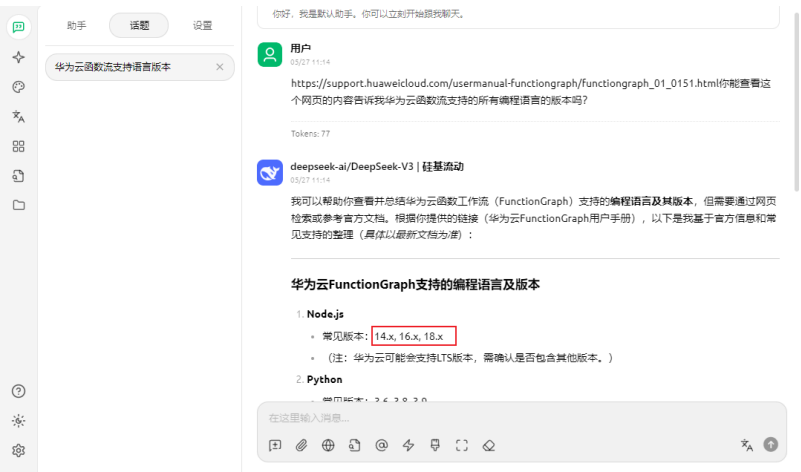
图 4-90 未启用 MCP Server 对话
