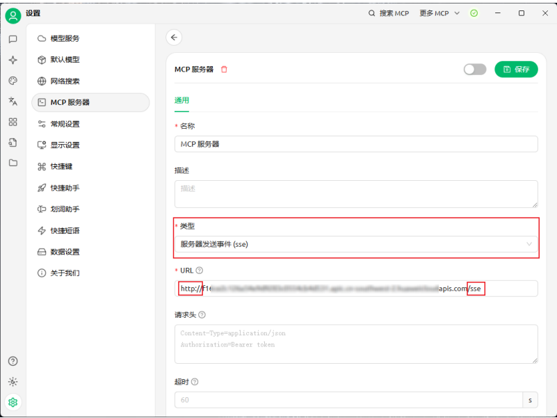
图 4-89 配置 MCP 服务器
