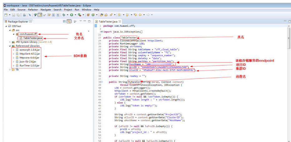
图 3-12 样例代码说明
