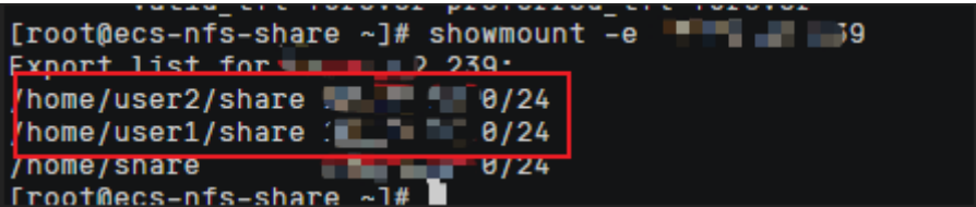
图 4-58 查看共享信息
