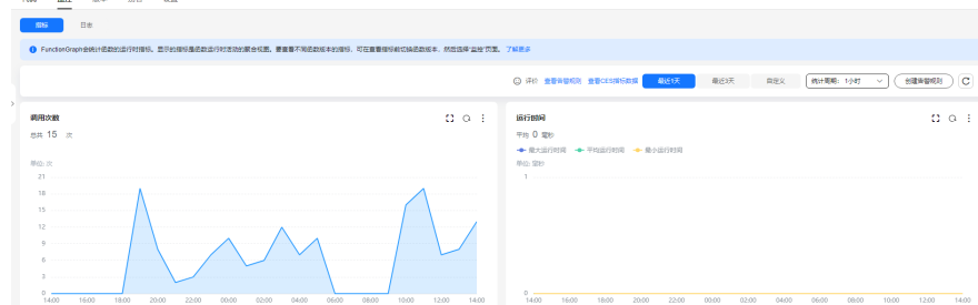
图 3-5 函数指标
