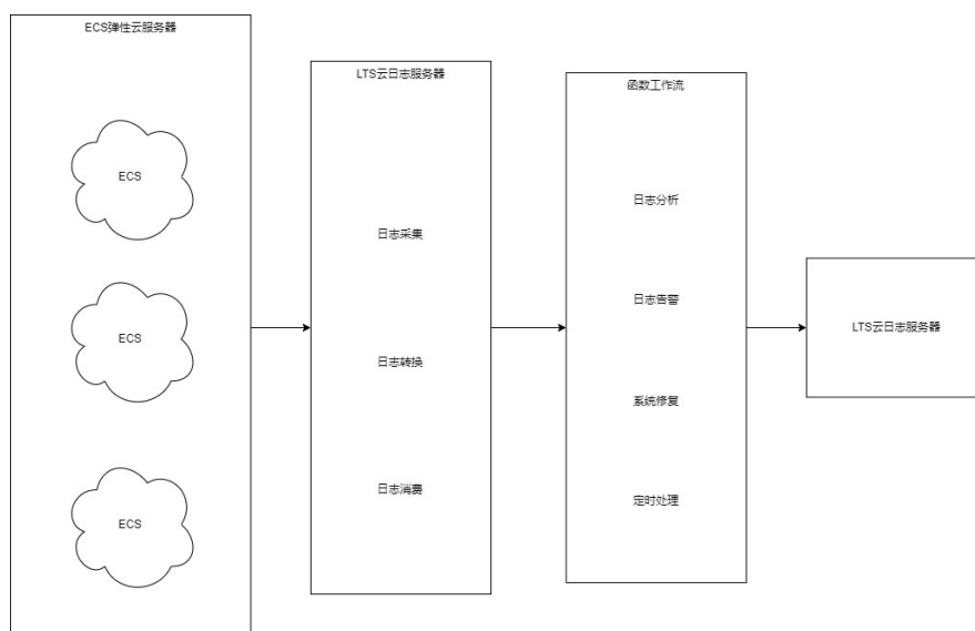
图 2-49 处理流程
