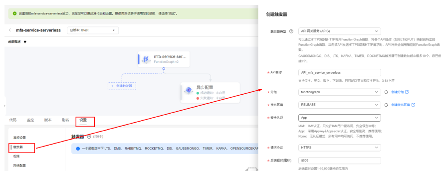
图 4-47 创建触发器
