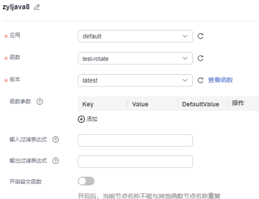
图 2-64 配置元信息
