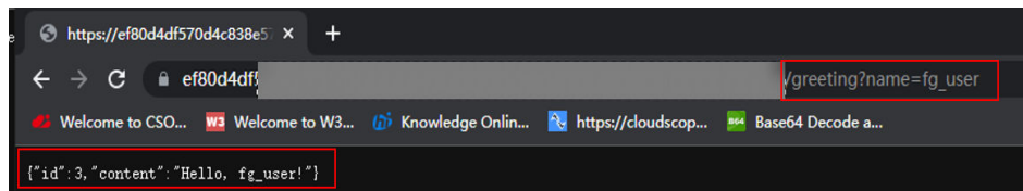
图 4-6 调用函数
