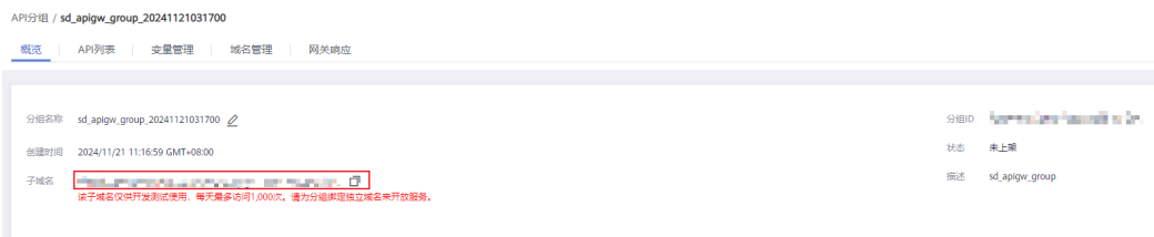
图 3-26 复制子域名
