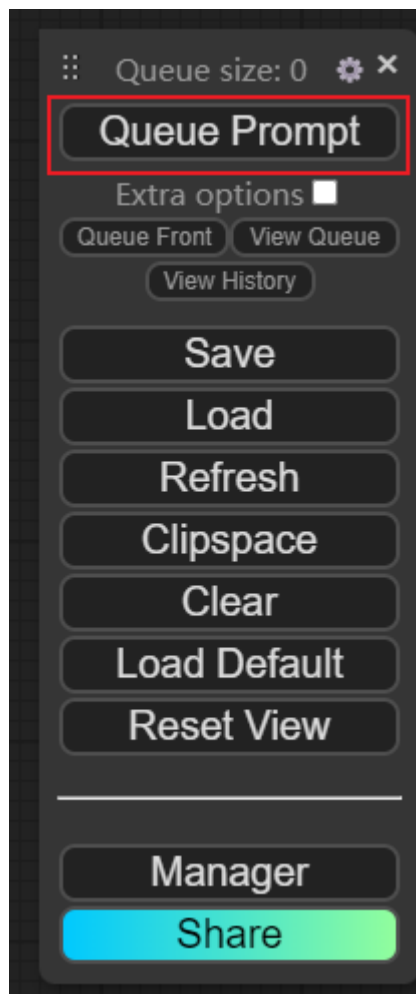
图 3-53 生成图像
