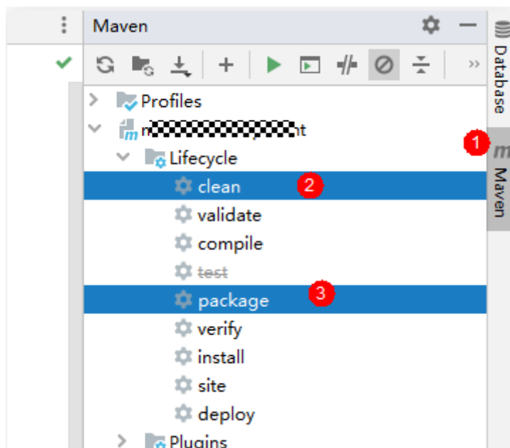
图 4-31 IDEA 打包
