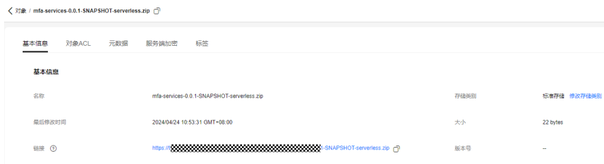
图 4-36 对象地址
