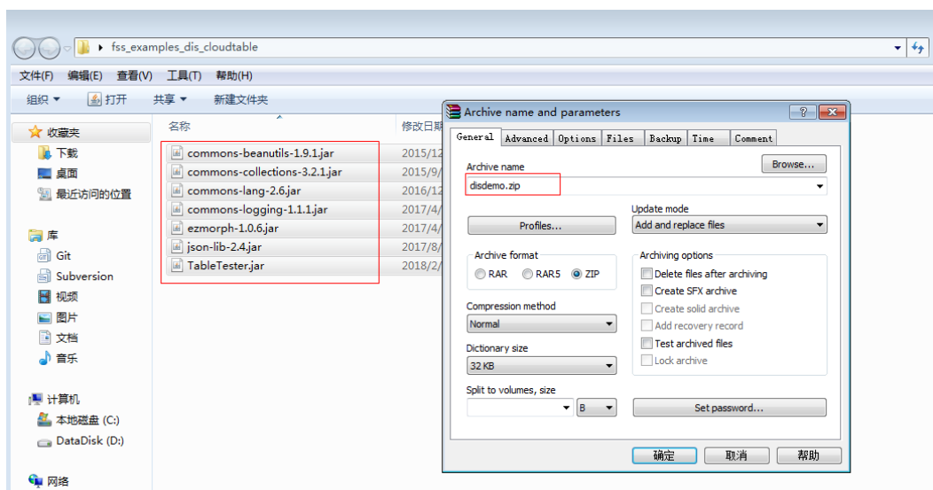
图 2-22 打 ZIP 包
