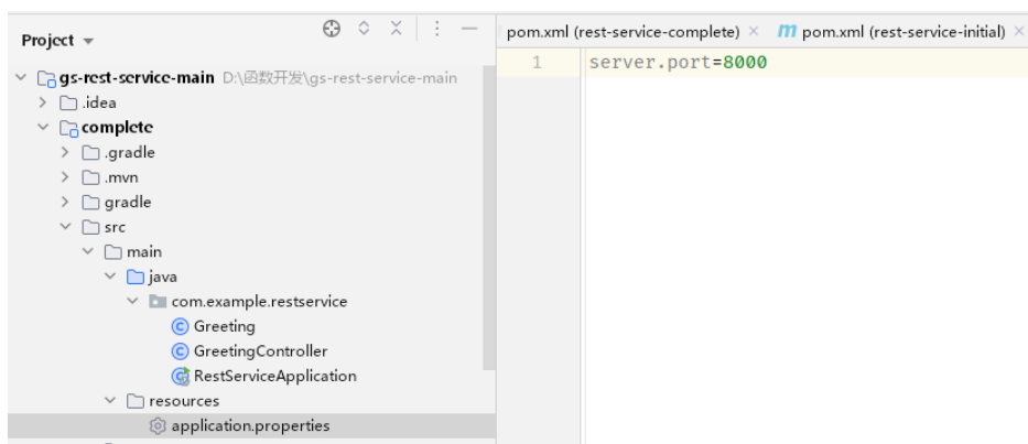
图 4-2 配置 8000 端口
