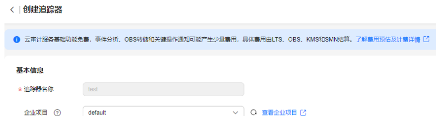
图 3-2 配置追踪器
