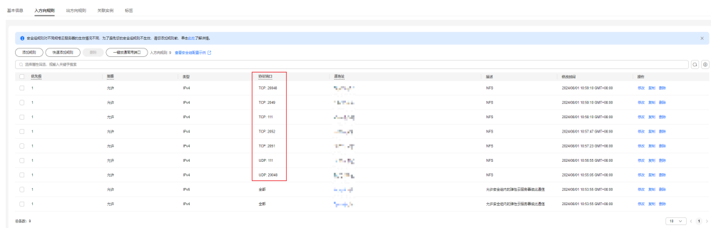
图 3-38 安全组设置
