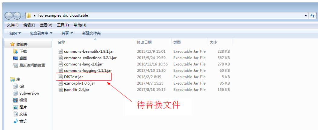
图 2-20 文件目录
