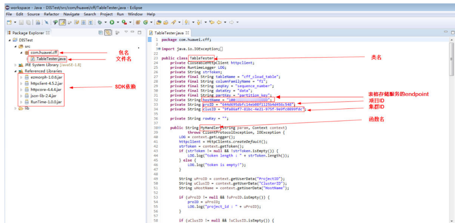
图 2-13 样例代码说明
