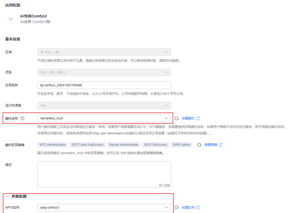
图 3-55 AI 绘画 ComfyUI 应用配置
