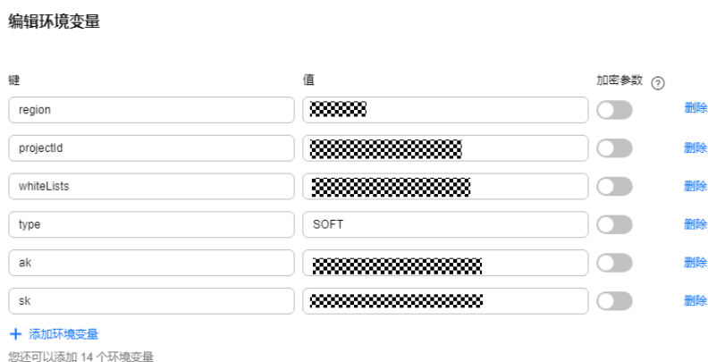
图 3-8 配置环境变量
