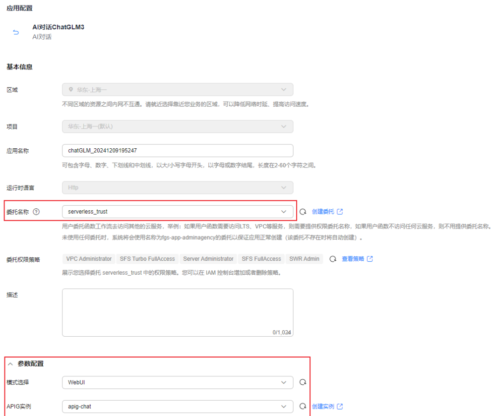
图 3-71 AI 对话 ChatGLM3 应用配置
