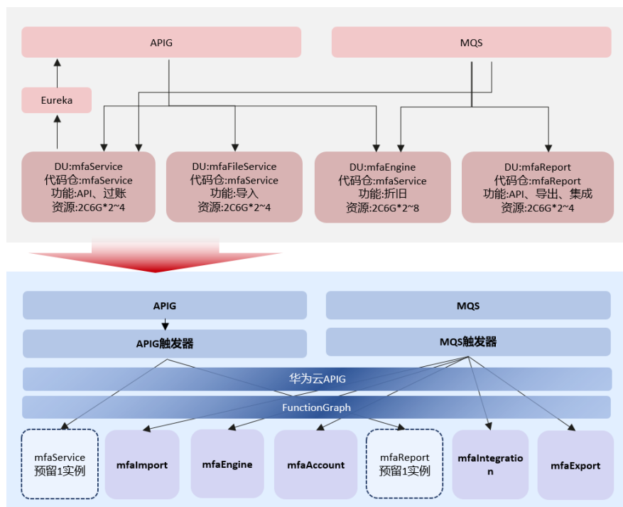
图 4-22 MFA Serverless 改造前后架构
