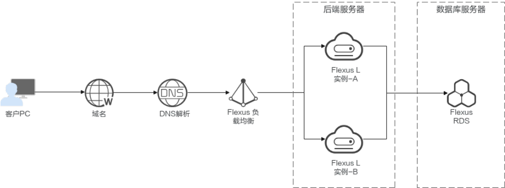
图 6-1 使用 Flexus L 实例部署高可用架构应用集群架构图
