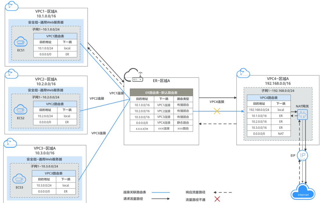
图 9-3 同区域 VPC 共享 SNAT 组网规划
