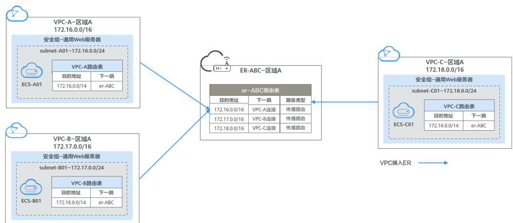
图 10-5 迁移完成后组网示意图
