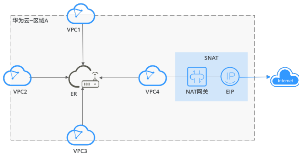
图 9-1 VPC 共享 SNAT
