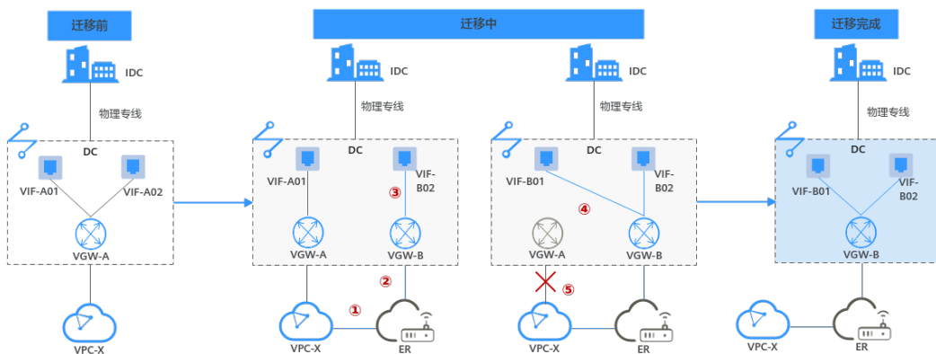
图 11-1 DC 直连 VPC 组网迁移架构图
