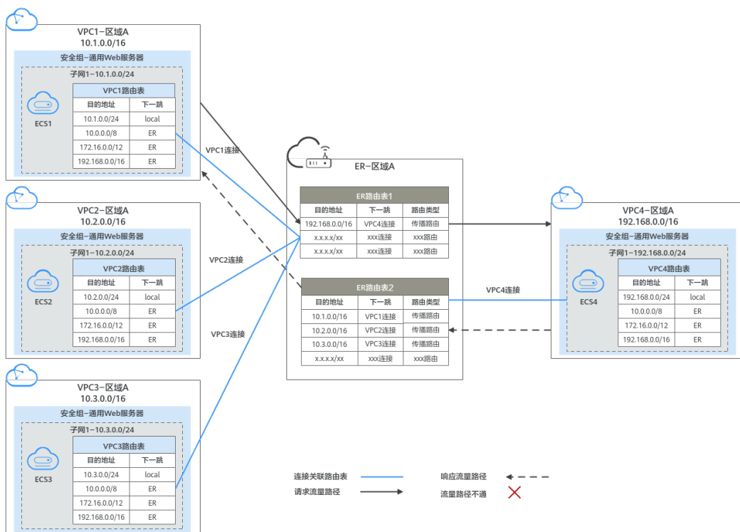
图 3-3 同区域 VPC 隔离组网规划
