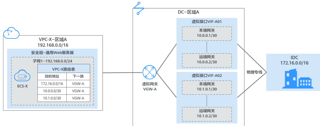
图 11-2 迁移前组网示意图
