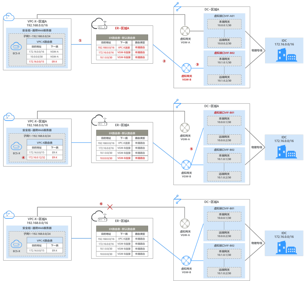
图 11-3 迁移中组网示意图
