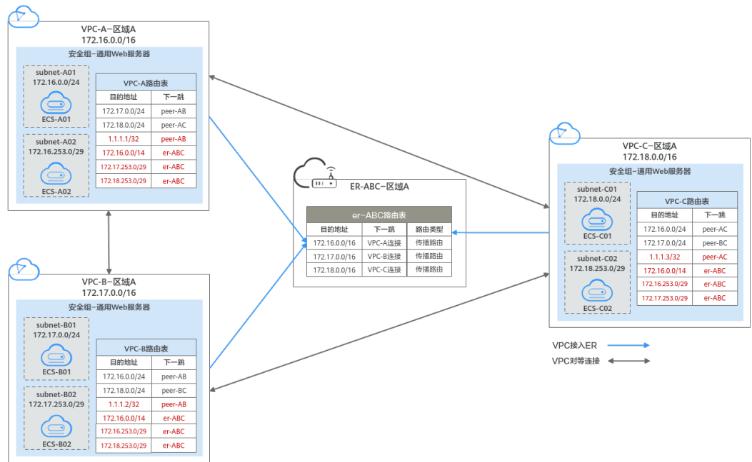
图 10-4 迁移中组网示意图
