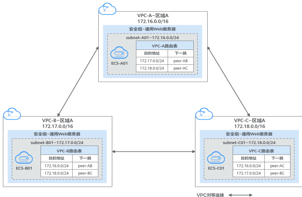
图 10-3 迁移前组网示意图
