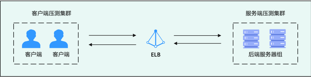
图 2-23 压测方案架构
