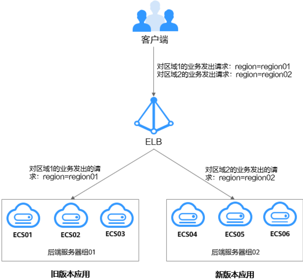
图 6-9 基于查询字符串实现新旧版本应用平滑过渡
