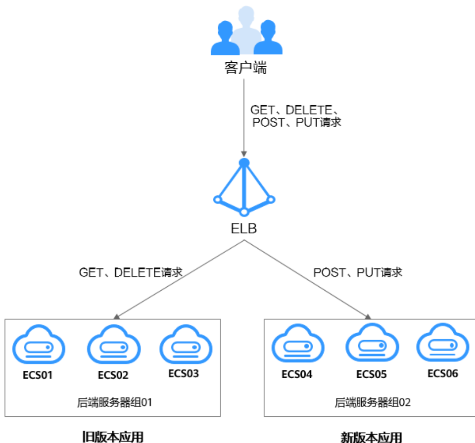
图 6-3 基于 HTTP 请求方法实现新旧版本应用平滑过渡
