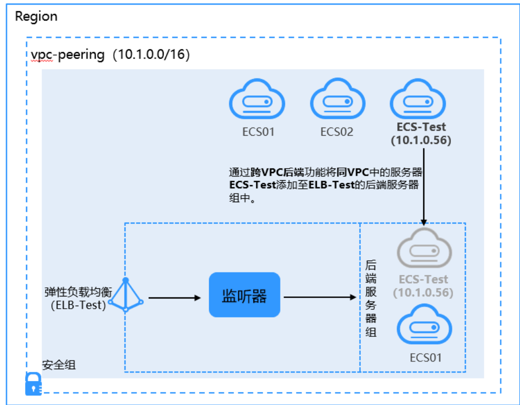
图 2-14 使用 IP 类型后端功能添加同 VPC 的 ECS 至 ELB
