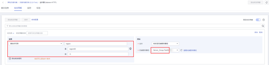
图 6-11 基于查询字符串将部分请求转发至新版本应用上
