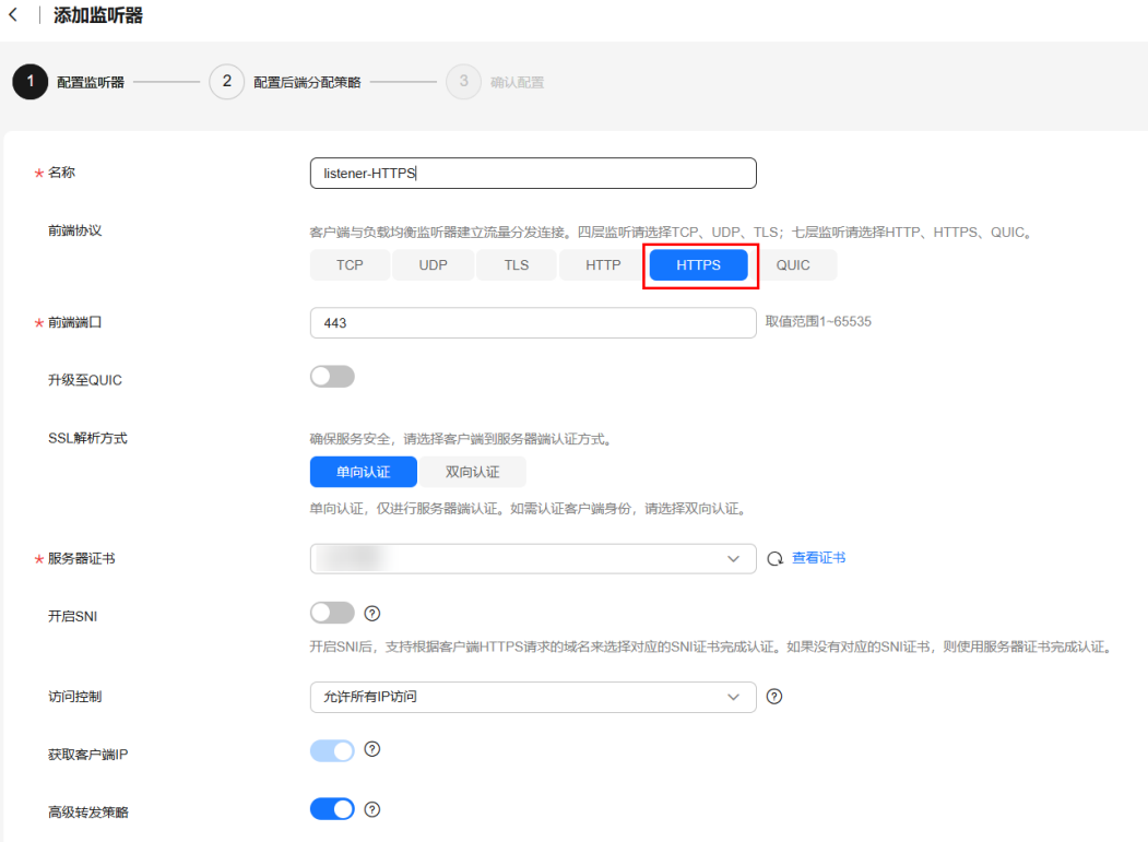
图 5-6 添加 HTTPS 监听器并配置单向认证
