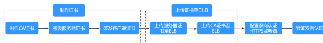
图 4-10 配置 HTTPS 业务双向认证操作流程
