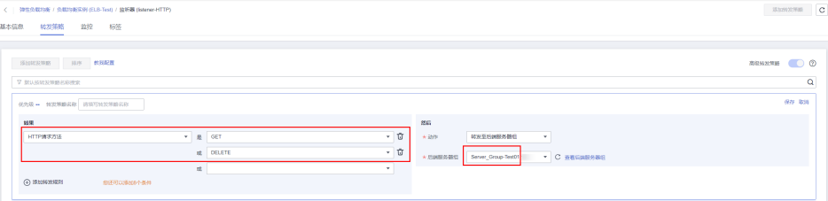
图 6-4 基于 HTTP 请求方法将部分请求转发至旧版本应用上
