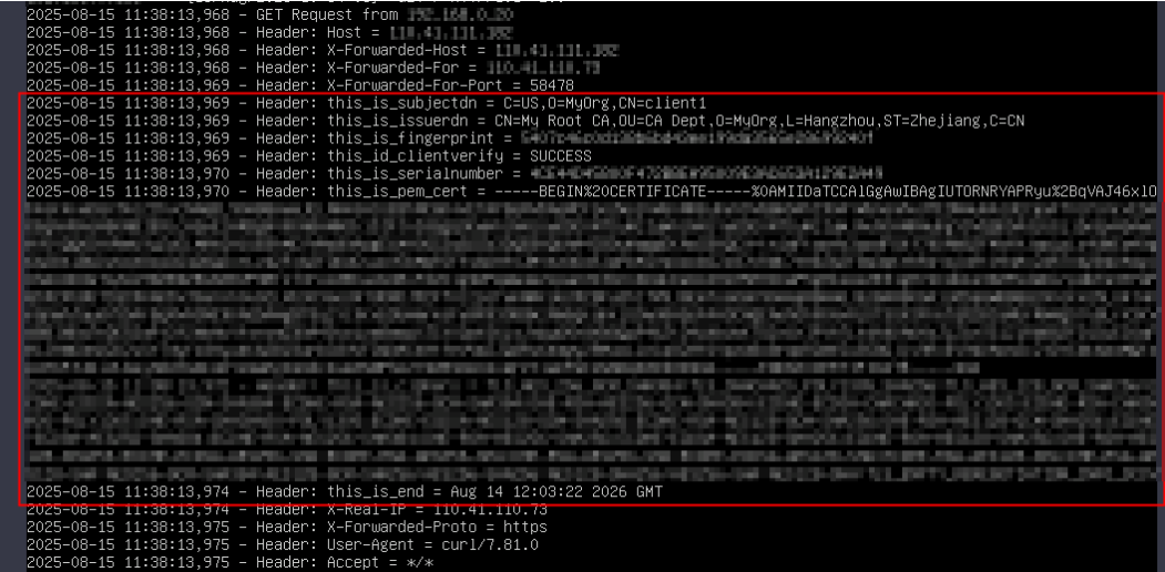
图 5-66 验证服务端获取到客户端证书信息
