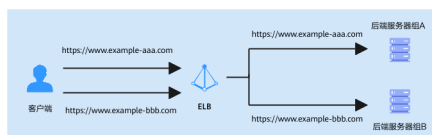
图 5-21 单 ELB 实例配置多域名业务转发示意图
