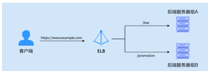
图 6-12 ELB 实例配置相同域名不同路径的业务转发示意图
