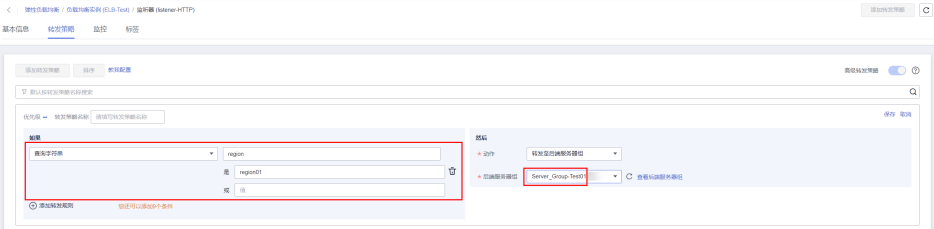
图 6-10 基于查询字符串将部分请求转发至旧版本应用上
