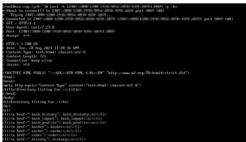
图 5-34 验证 Web 类服务应用的连通性
