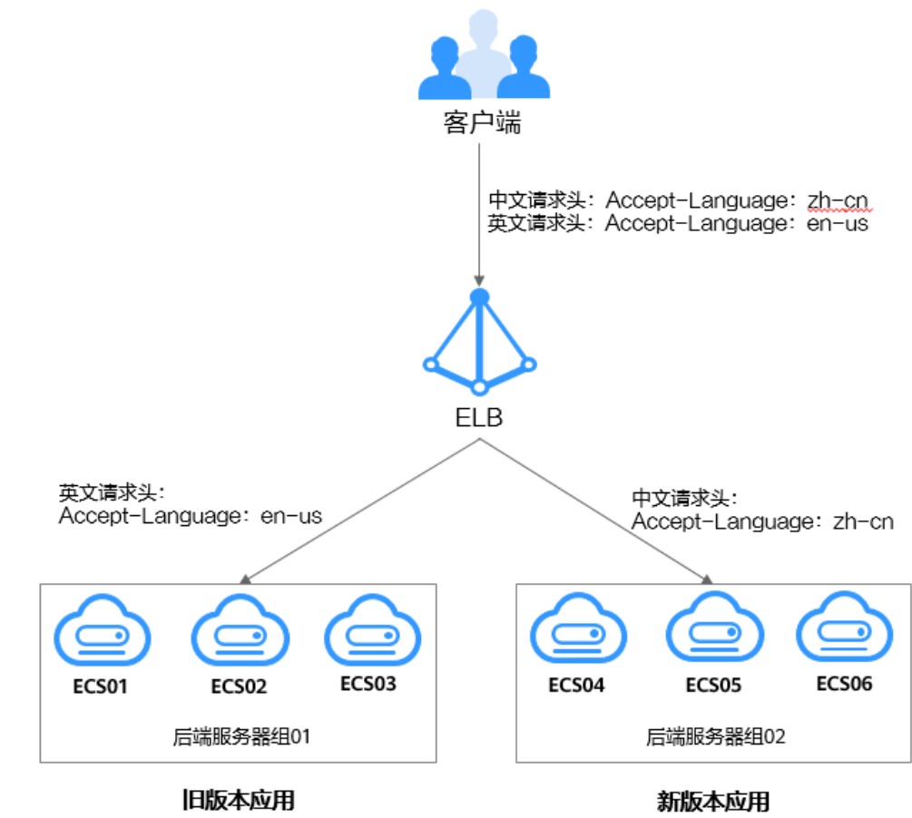
图 6-6 基于 HTTP 请求头实现新旧版本应用平滑过渡
