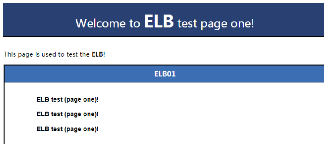
图 4-9 访问到 ECS01
