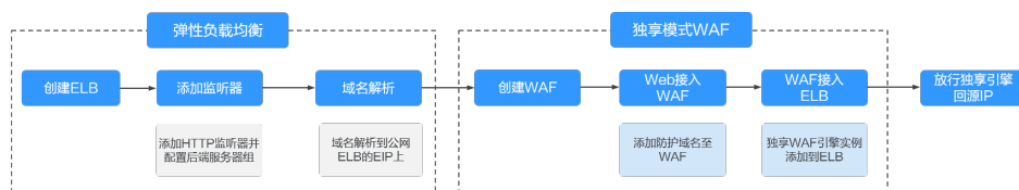
图 3-6 独享 WAF 接入应用型 ELB 的操作流程
