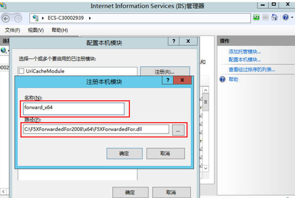
图 5-49 注册插件
