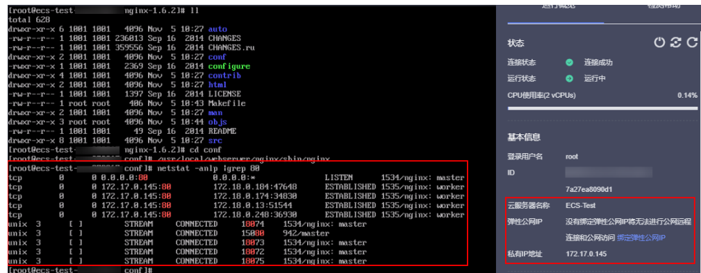
图 2-11 在 ECS-Test 上部署 Nginx
