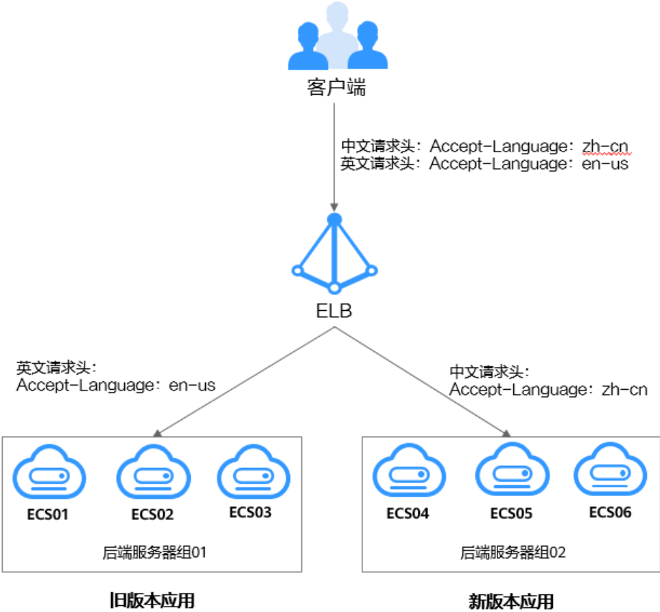
图 6-5 基于 HTTP 请求头实现新旧版本应用平滑过渡
