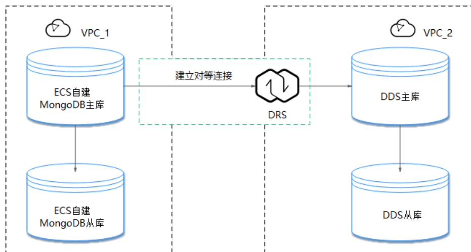
图 2-22 同区域不同 VPC 网络
