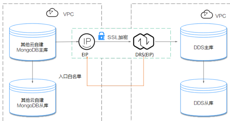
图 2-6 其他云自建 MongoDB 数据库实时迁移示意图
