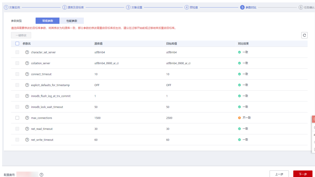
图 5-24 设置参数
