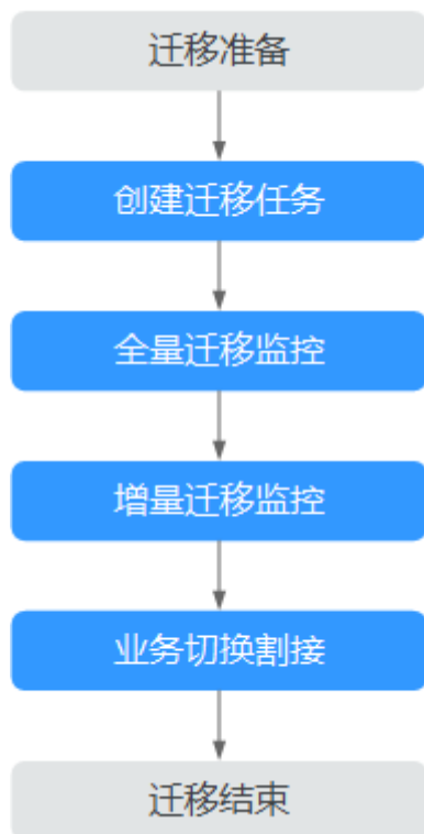
图 2-7 迁移流程图
