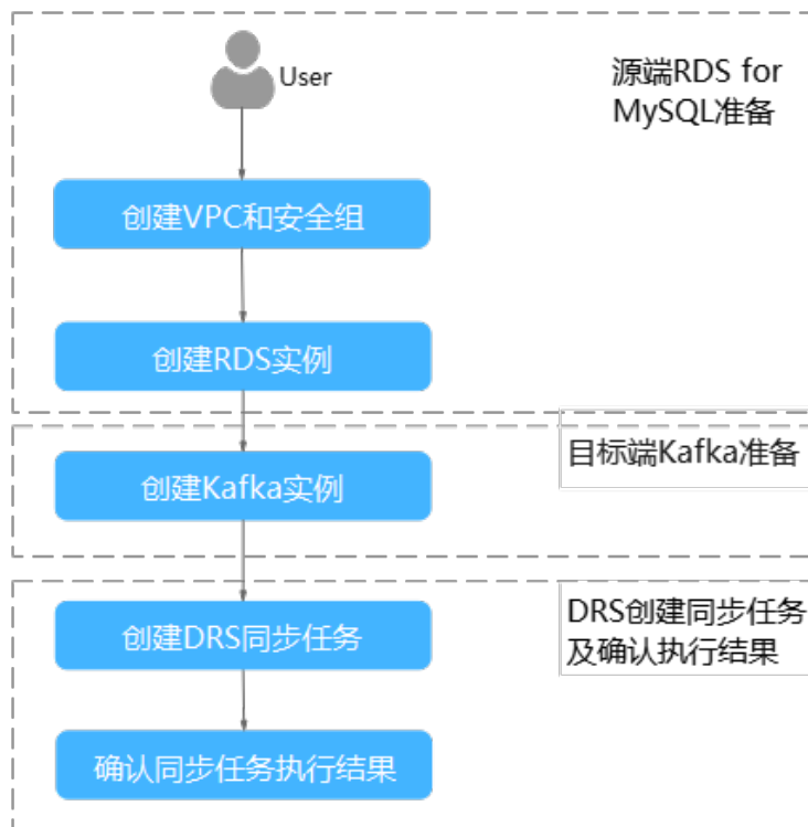
图 4-35 流程图
