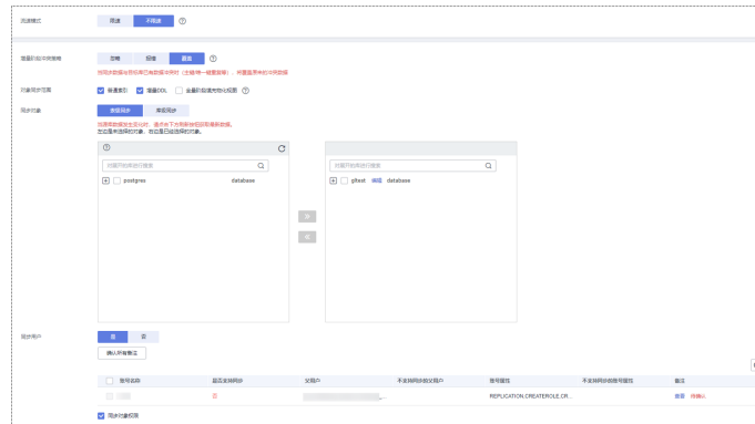
图 4-17 同步模式
