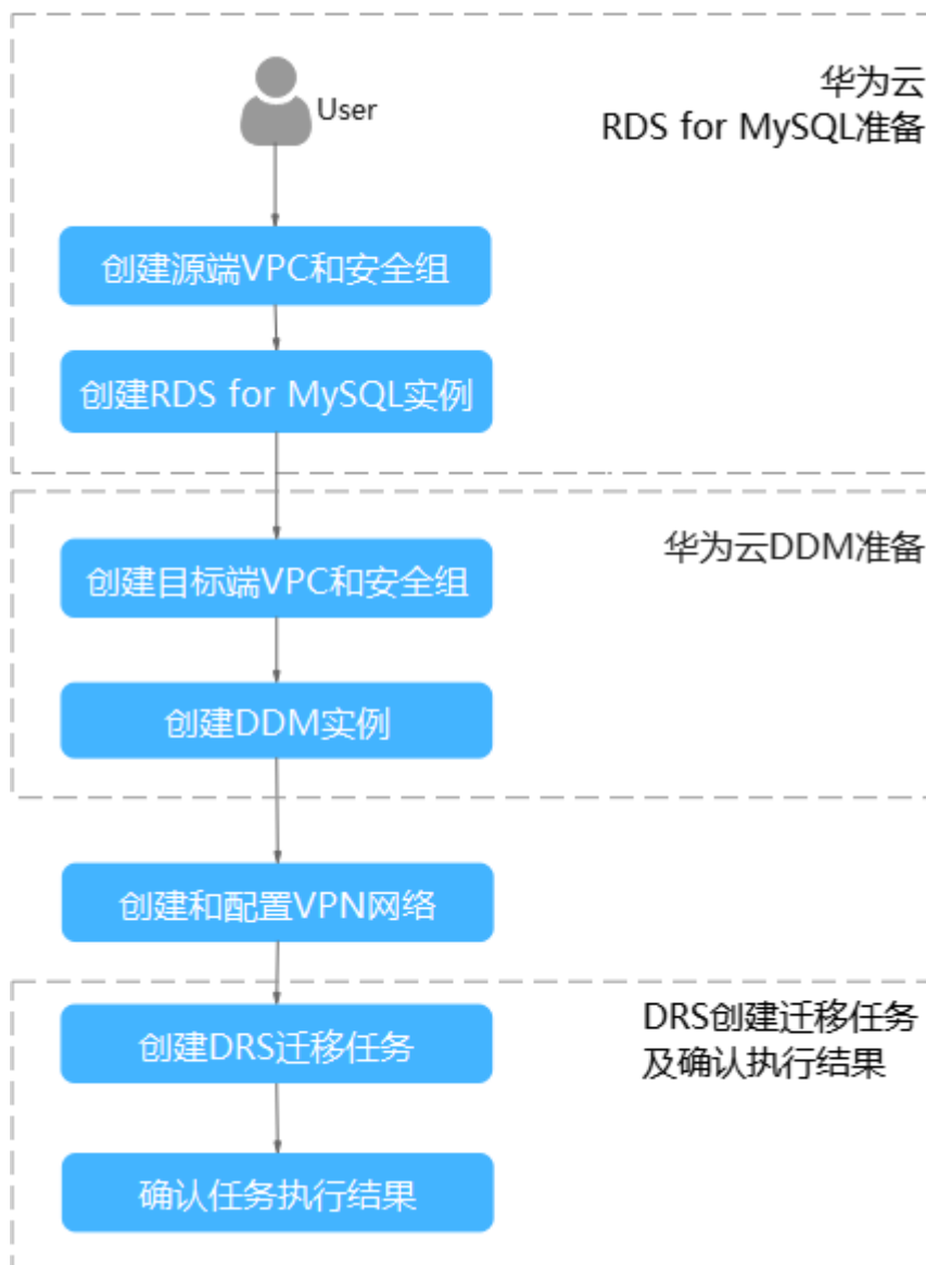
图 2-57 流程图
