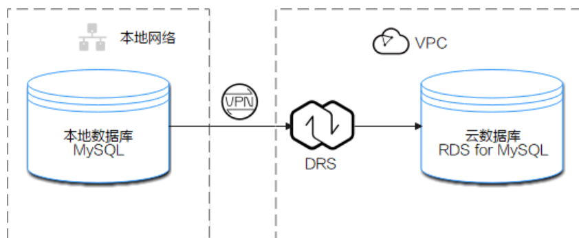
图 2-31 VPN 网络
