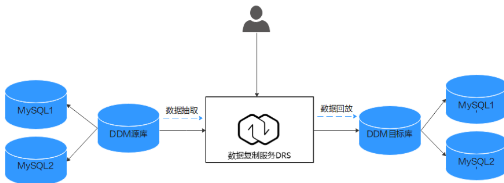
图 2-58 方案架构
