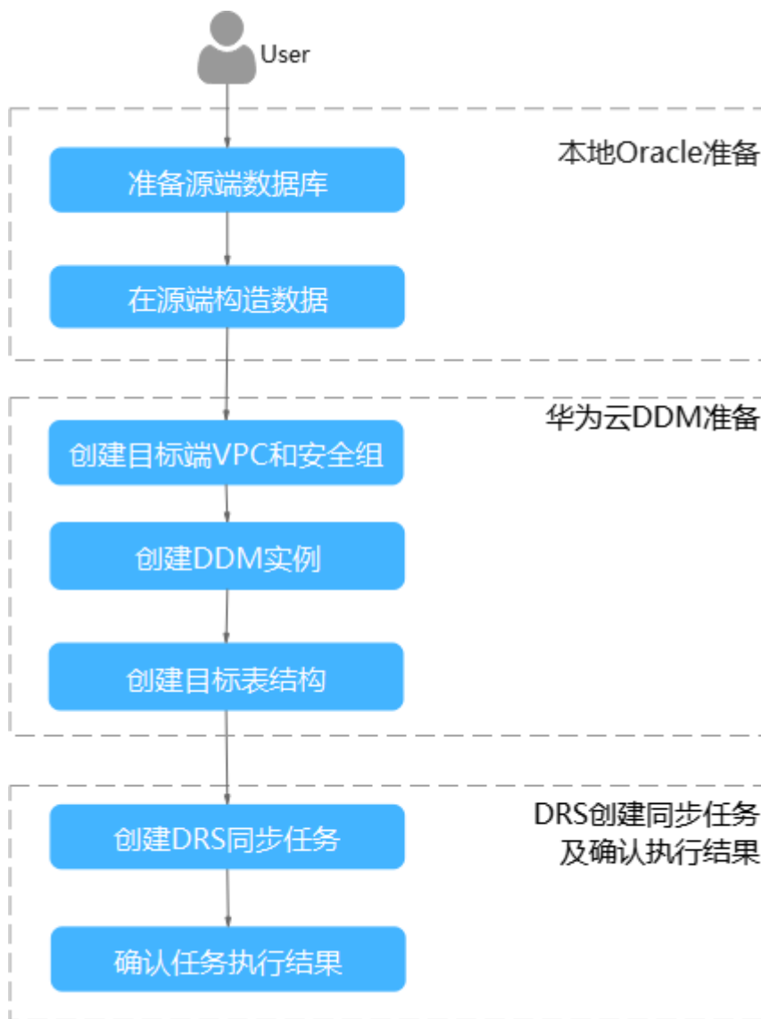
图 4-33 流程图
