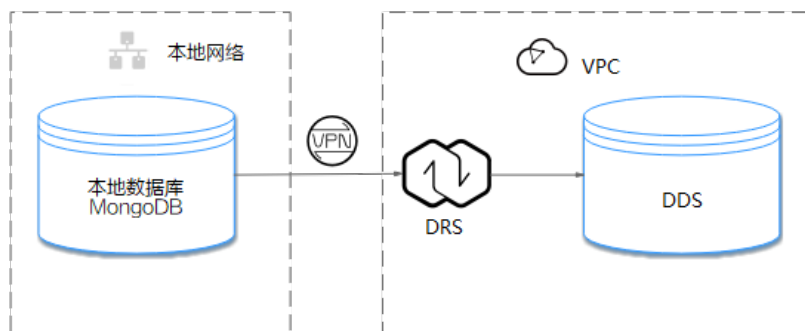
图 2-44 VPN 网络
