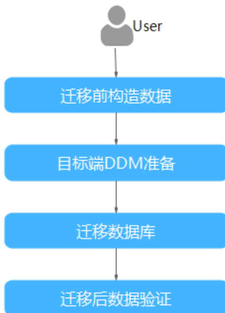
图 2-59 操作流程
