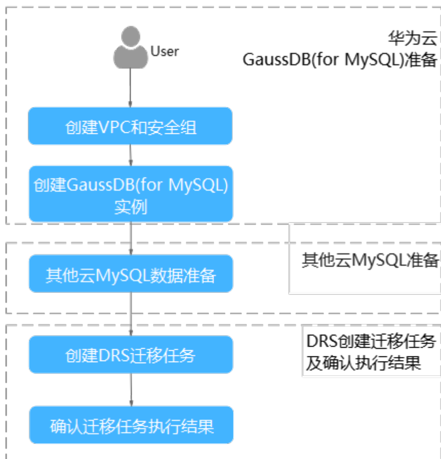
图 2-4 流程图
