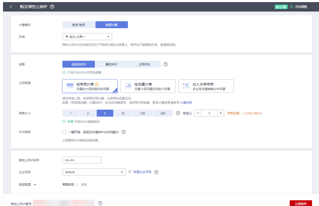
图 5-4 购买 EIP
