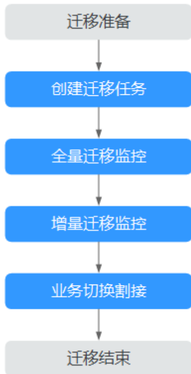
图 2-33 迁移流程图
