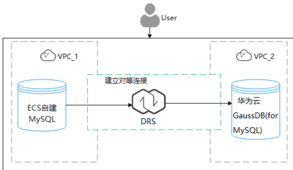
图 2-19 不同 VPC 场景的部署架构
