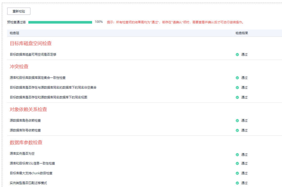
图 2-13 预检查
