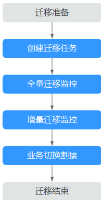
图 2-46 迁移流程图
