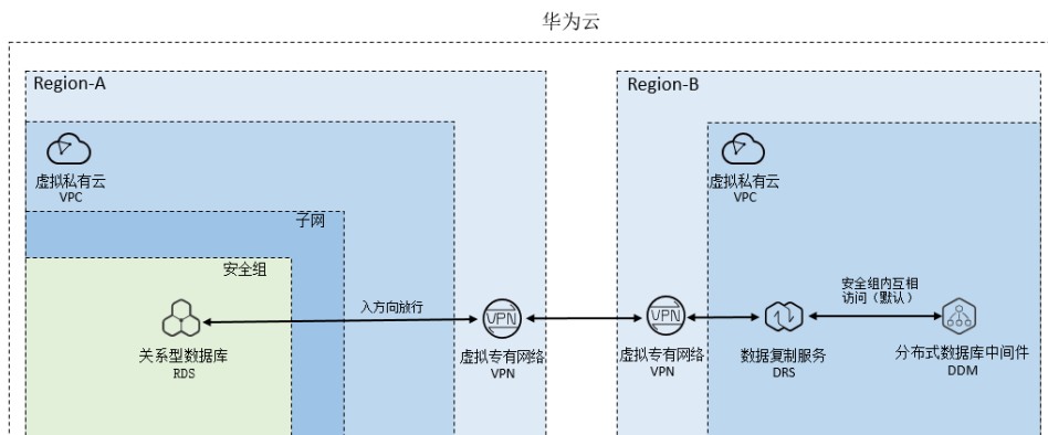
图 2-56 VPN 场景
