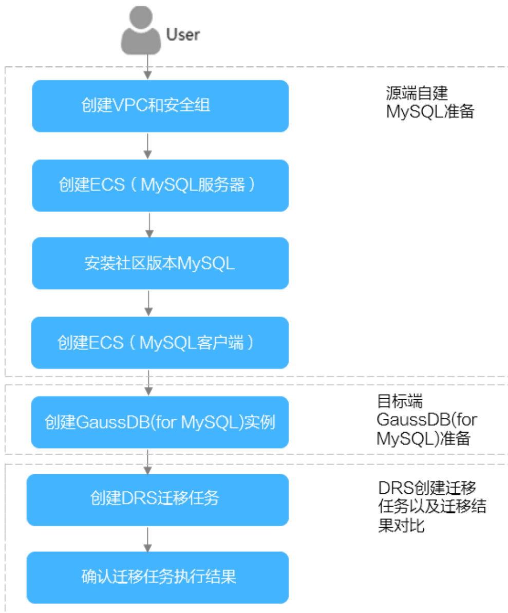
图 2-20 流程图
