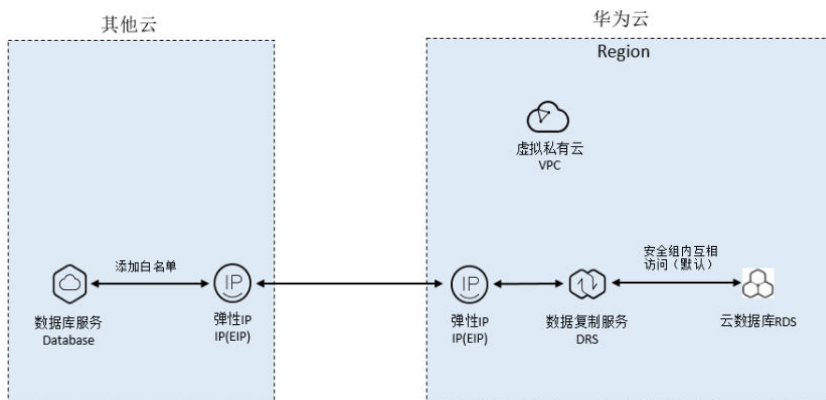
图 2-1 部署架构图
