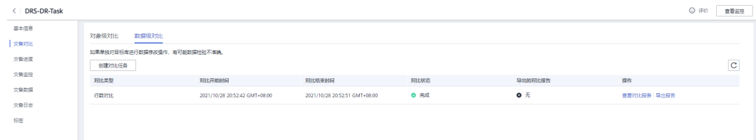
图 5-27 灾备对比
