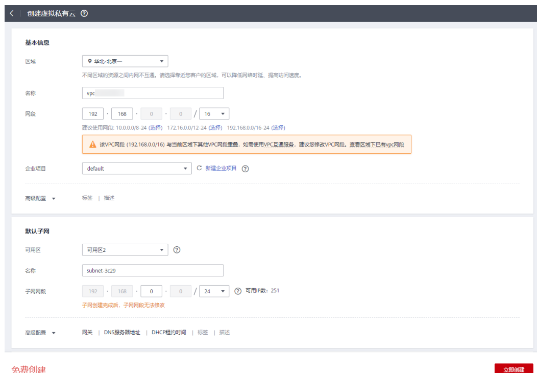
图 5-2 创建 VPC
