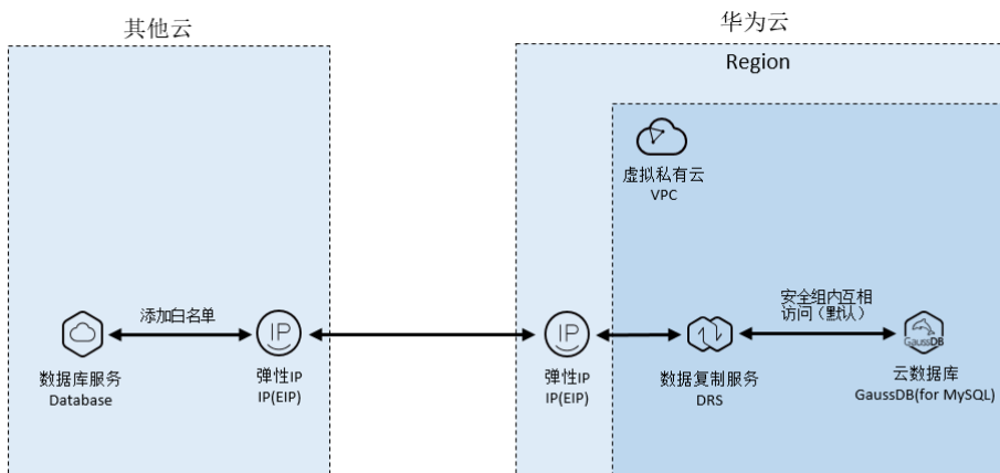
图 2-3 部署架构图
