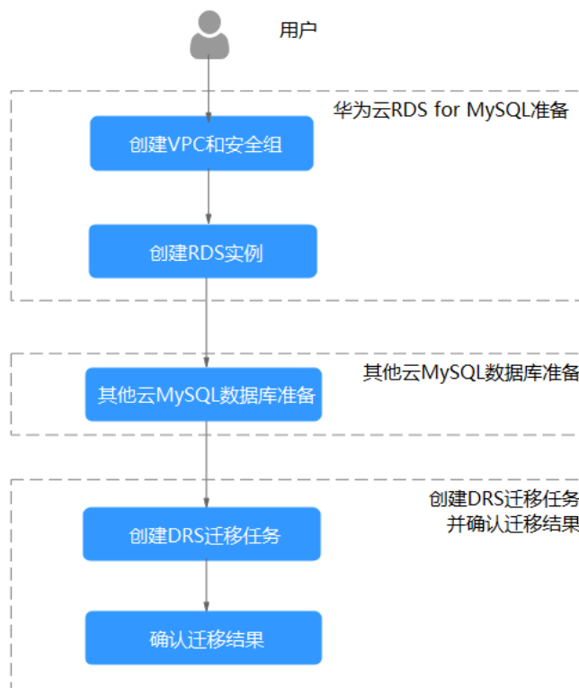
图 2-2 流程图
