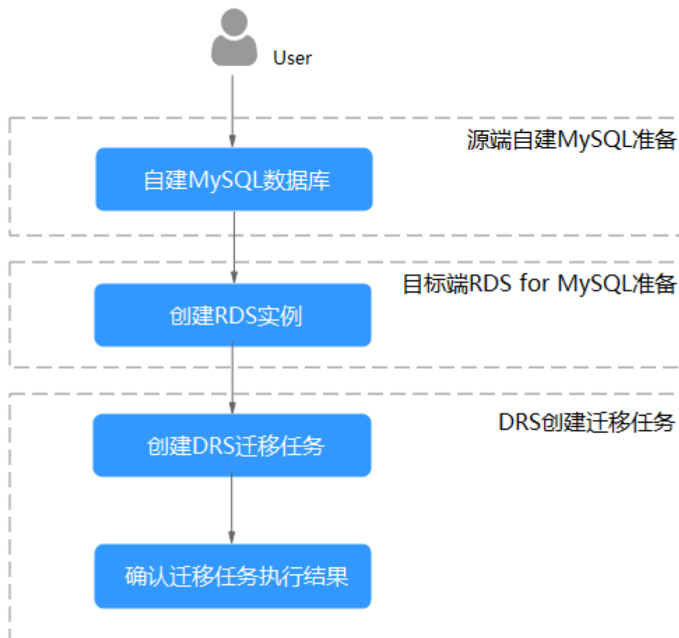
图 2-17 流程图
