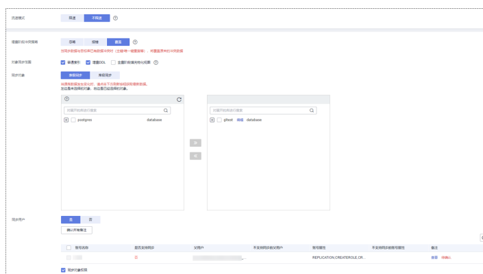
图 4-7 同步模式
