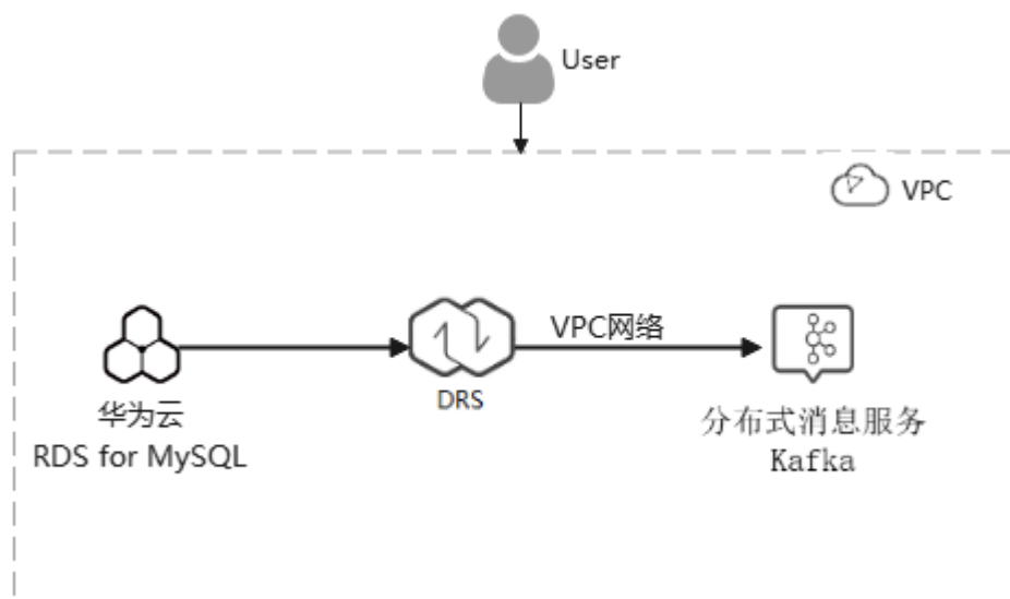
图 4-34 同 VPC 场景
