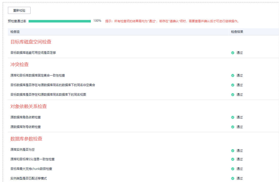
图 2-27 预检查
