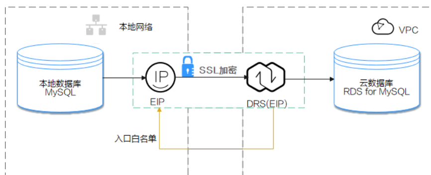
图 2-32 公网网络+SSL 安全连接
