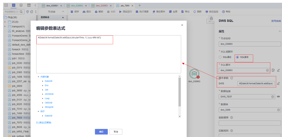
图 2-28 节点参数
