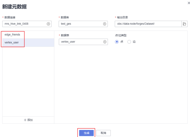
图 11-38 新建元数据
