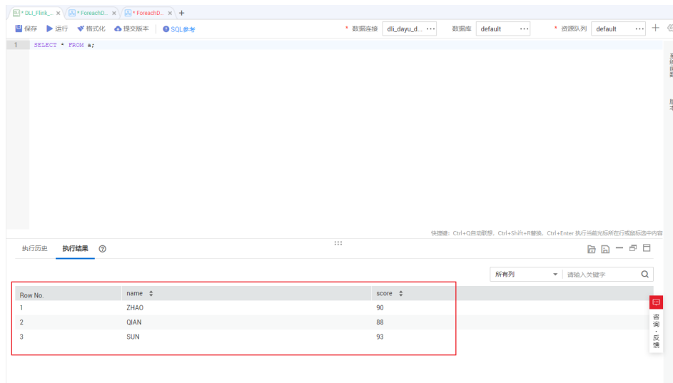
图 2-71 目的表数据
