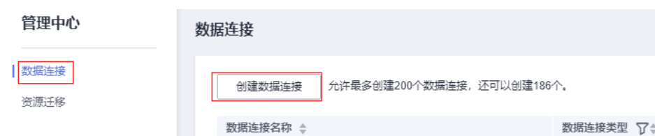
图 11-3 数据连接
