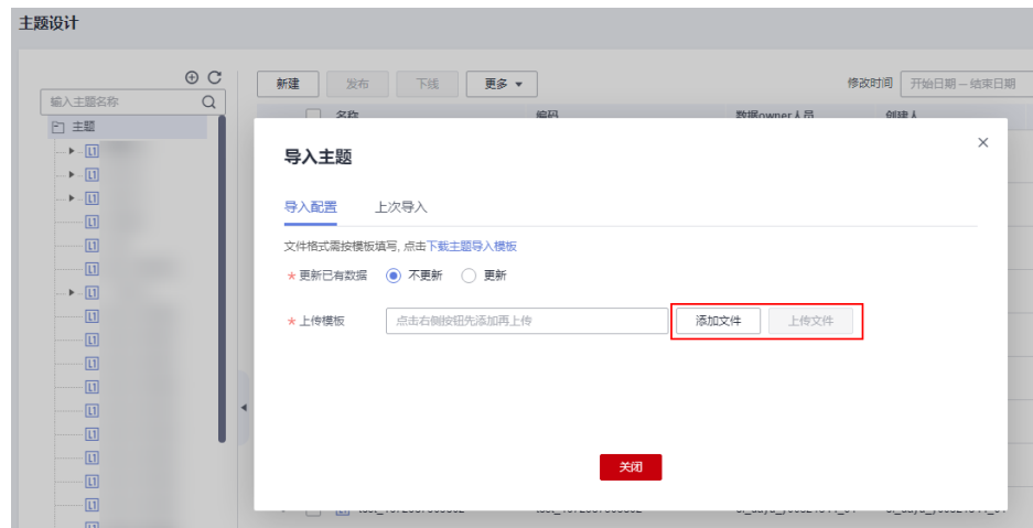
图 3-34 添加文件
