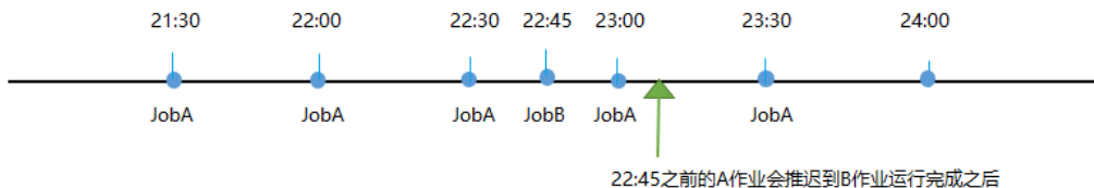
图 2-10 分钟依赖天
