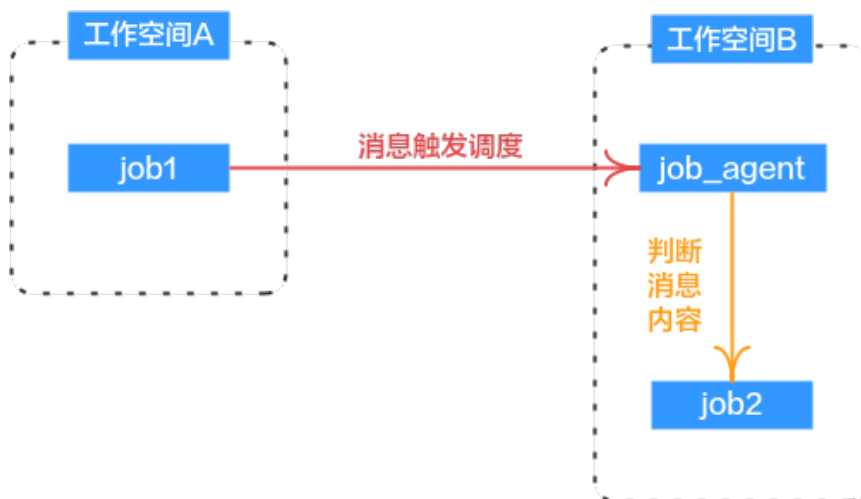
图 2-76 调度方案
