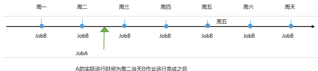
图 2-20 周依赖天
