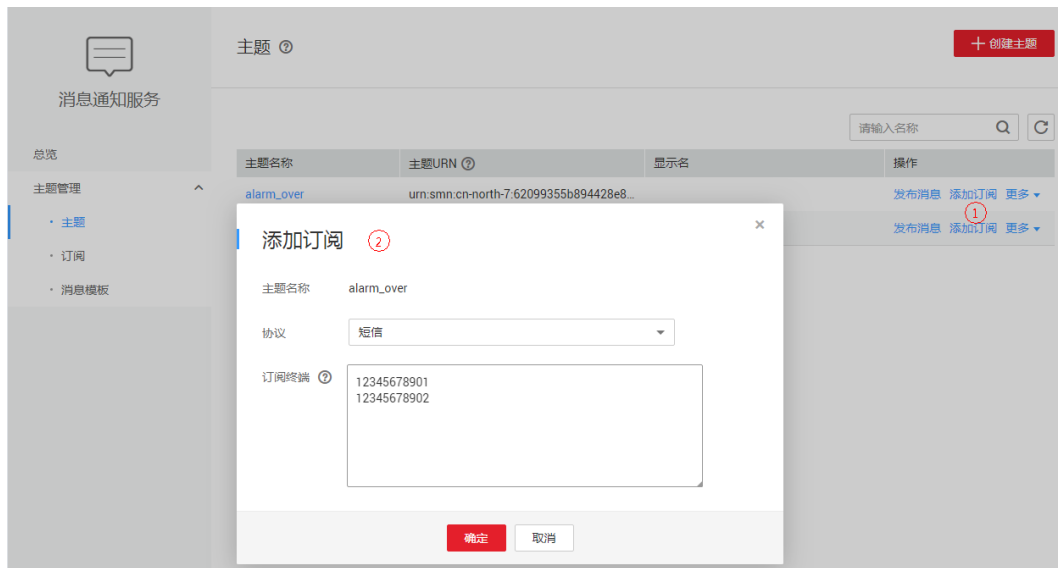
图 14-6 添加订阅
