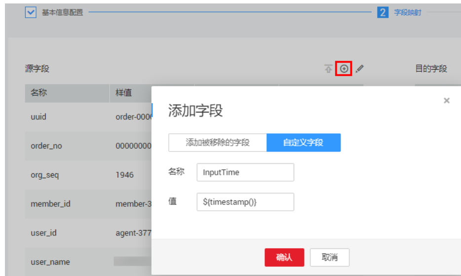
图 1-18 添加字段
