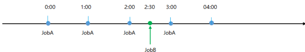
图 2-14 小时依赖天
