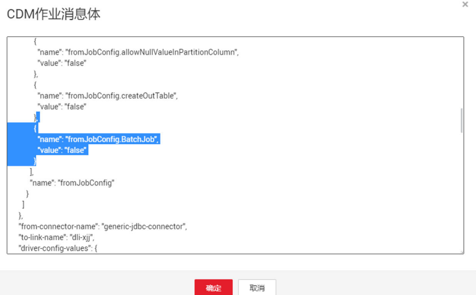
图 10-12 修改属性
