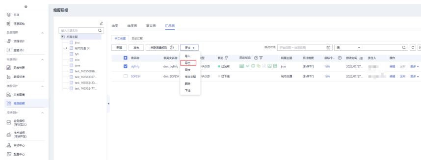
图 3-30 导出汇总表
