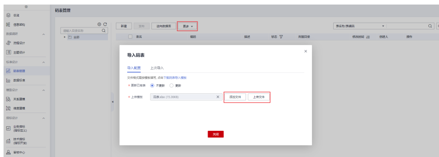
图 3-36 导入码表
