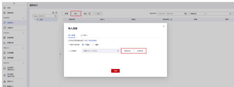
图 3-31 导入流程
