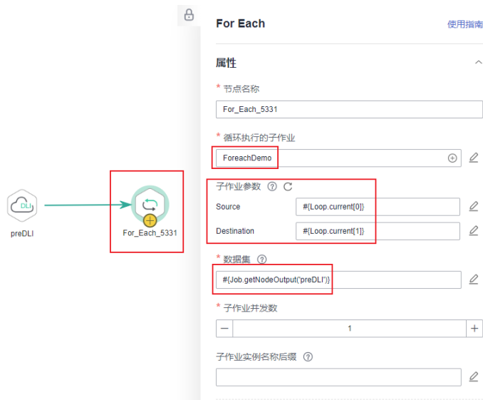
图 2-69 配置 For Each 节点
