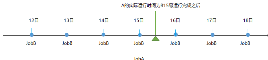
图 2-23 月依赖天
