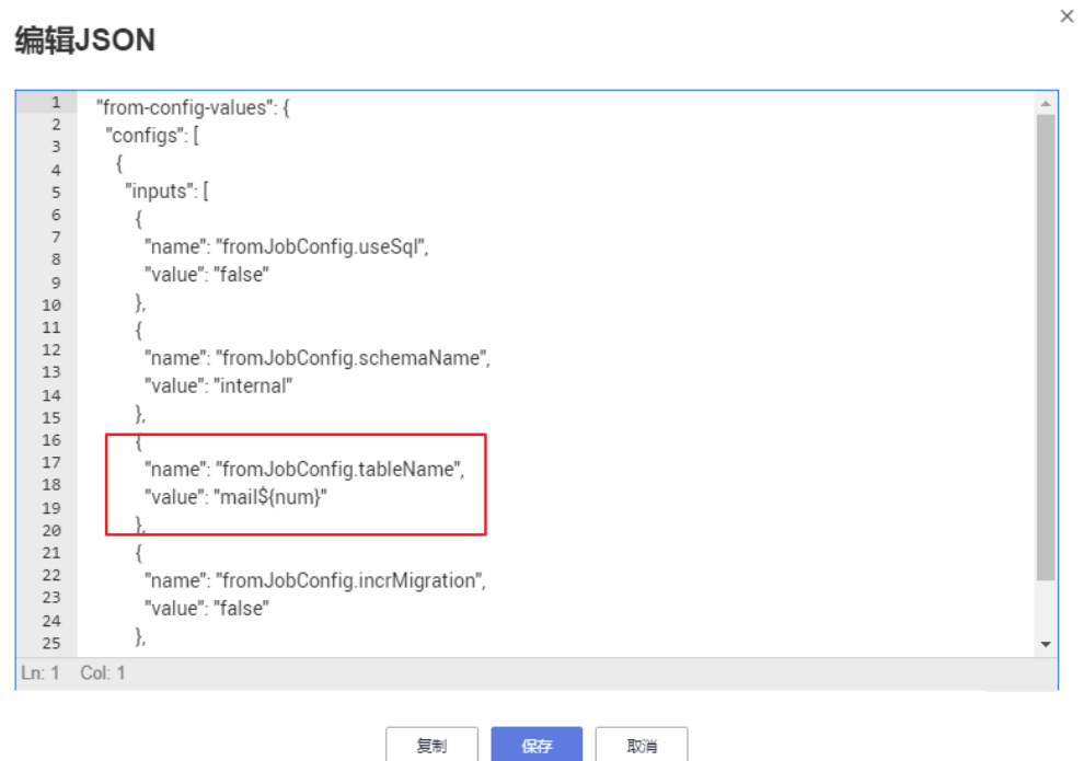
图 10-7 编辑 JSON
