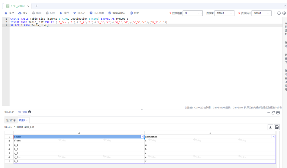
图 2-64 Table_List 表数据
