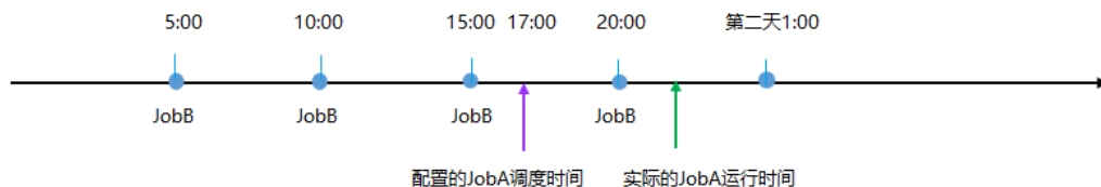
图 2-16 天依赖小时
