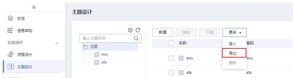
图 3-20 导出主题
