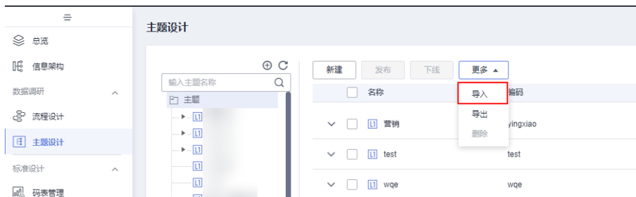
图 3-33 导入主题
