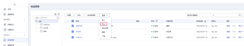
图 3-21 导出码表
