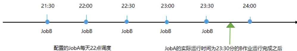
图 2-15 天依赖分钟
