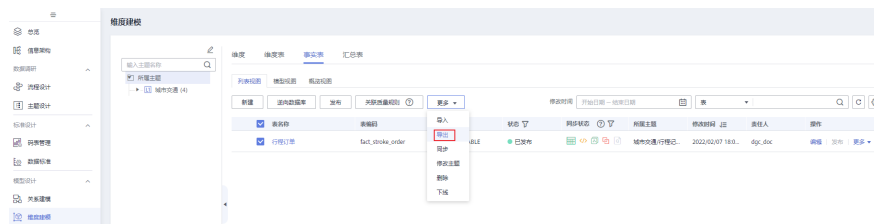
图 3-27 导出事实表
