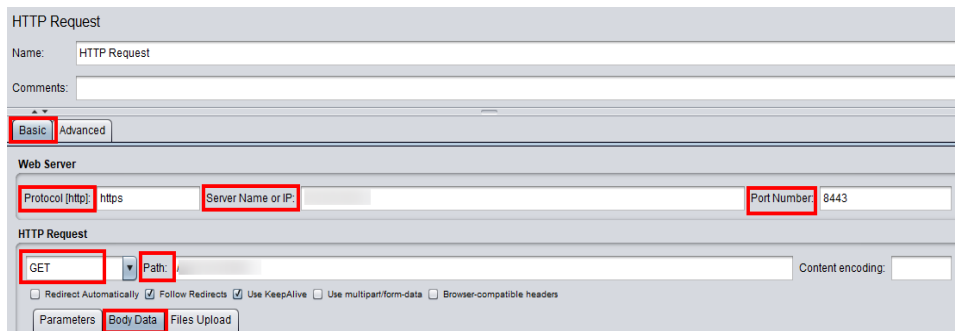
图 3-4 Basic 页签配置
