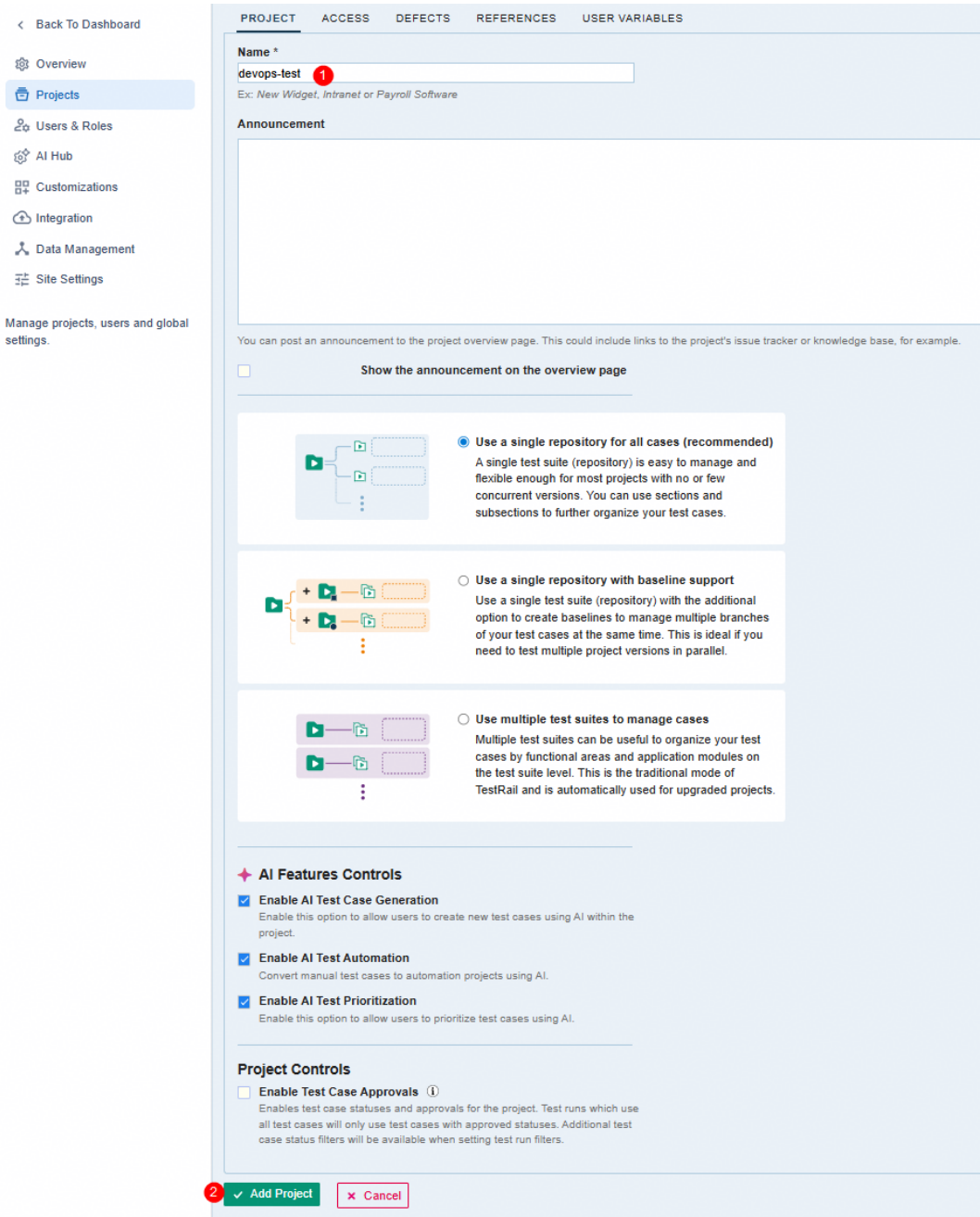
图 7-6 在 TestRail 创建项目
