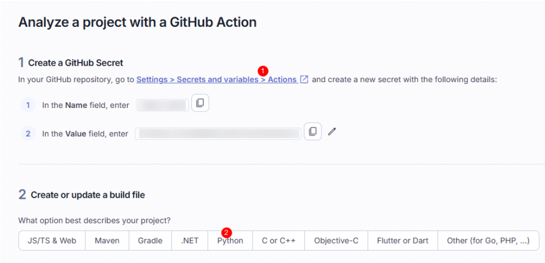
图 7-11 对接 GitHub Actions 的配置参数
