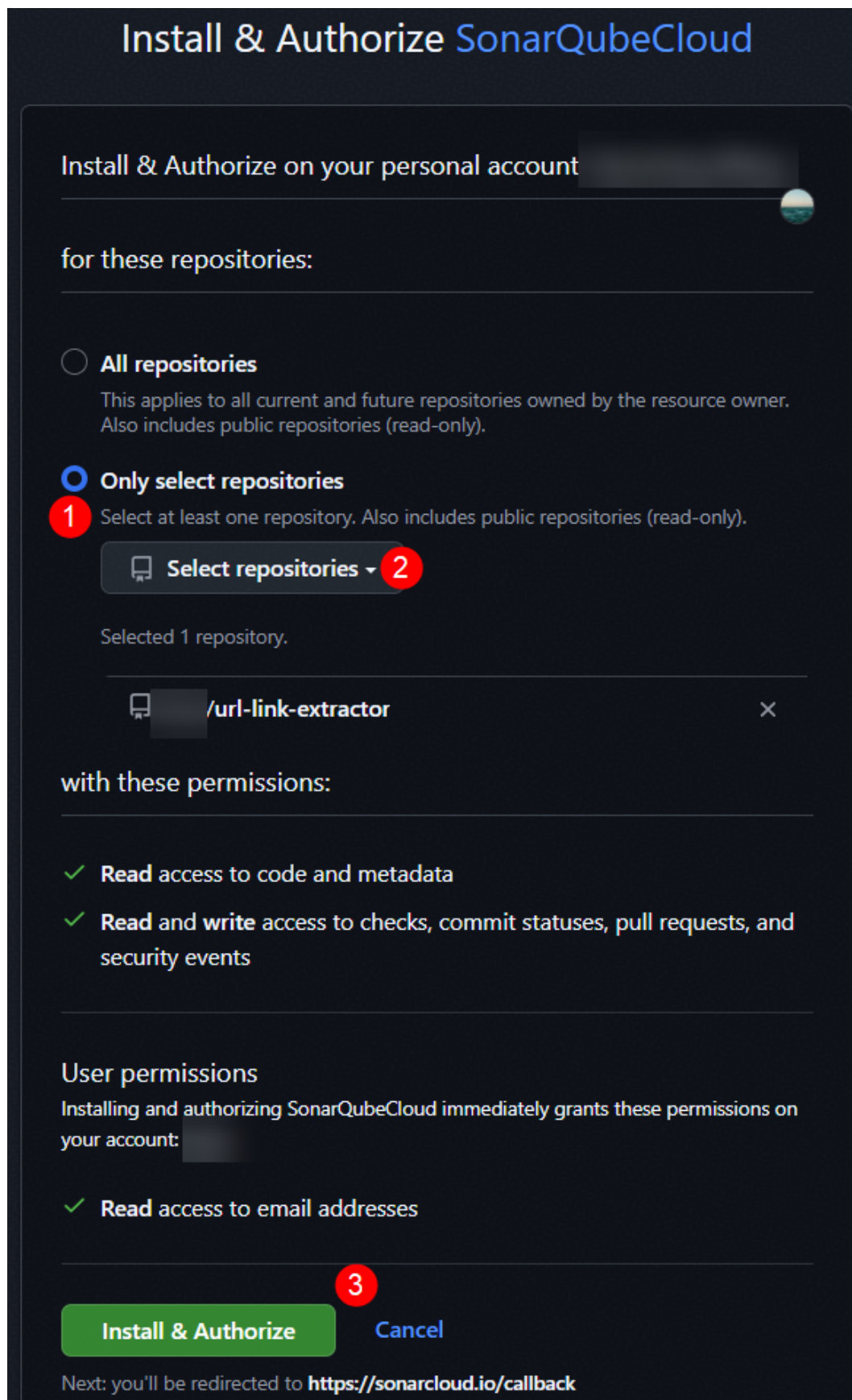
图 7-7 选择需要检查的代码仓
