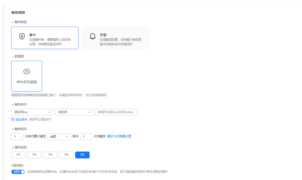
图 1-8 触发规则
