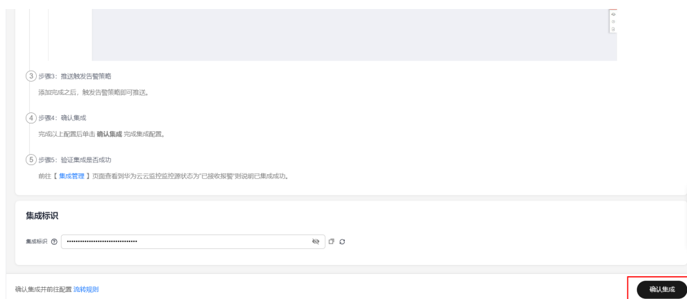
图 1-6 确认集成
