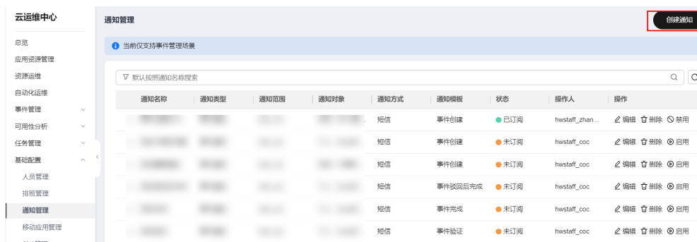
图 1-11 创建通知
