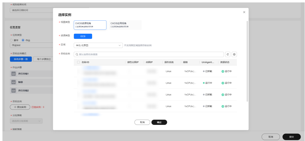
图 3-28 选择实例
