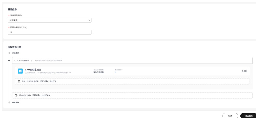
图 2-18 完成配置
