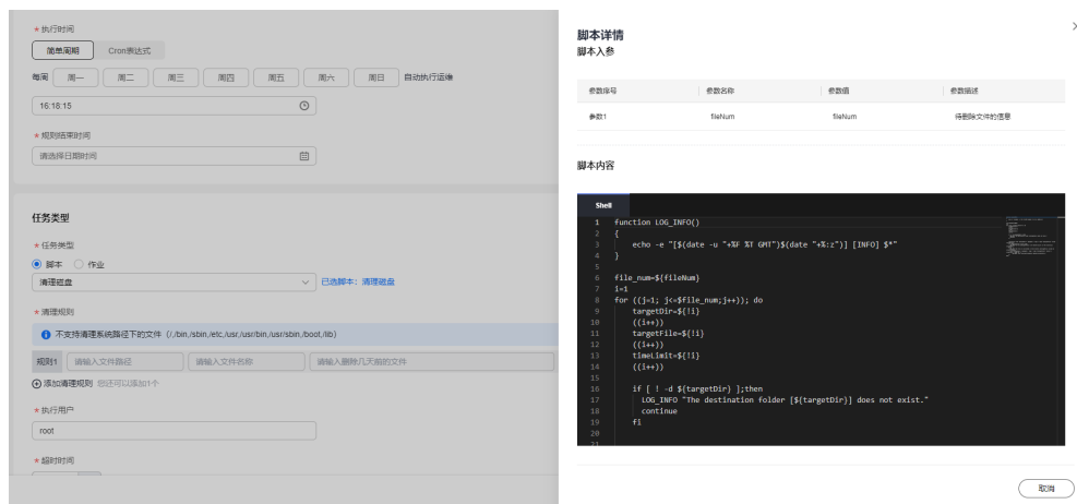
图 3-24 脚本详情
