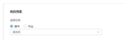
图 1-9 响应预案
