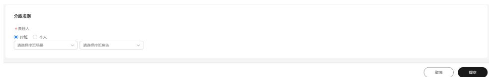
图 1-10 分派规则
