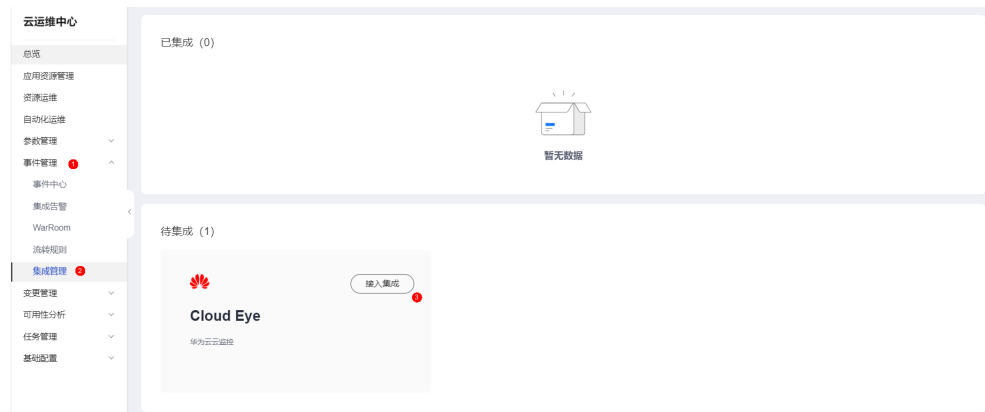
图 1-2 接入集成
