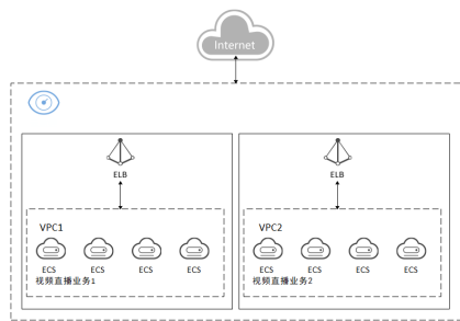
图 6-2 视频直播业务架构图
