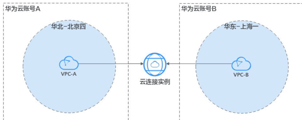
图 1-6 通过云连接实例实现跨区域跨账号 VPC 互通组网
