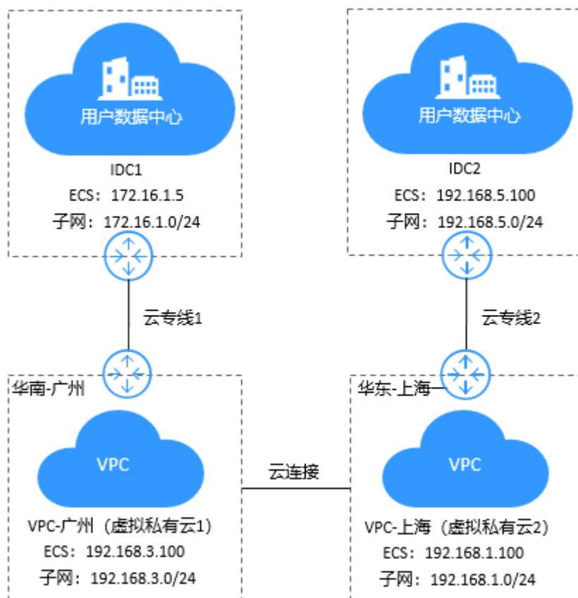
图 1-10 逻辑互联示意图
