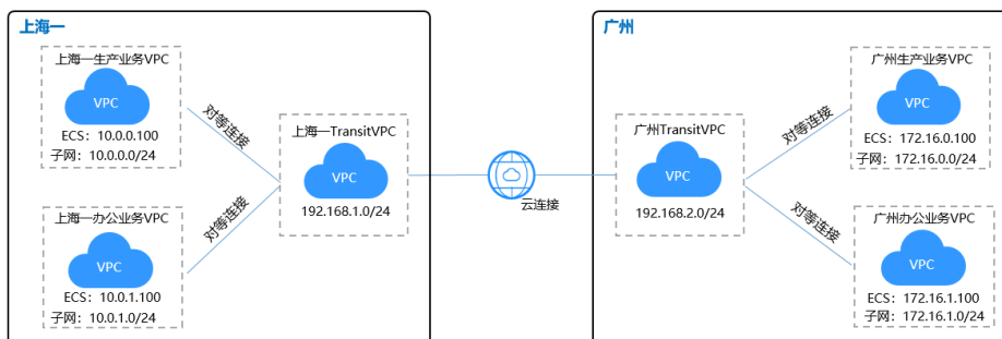
图 1-24 逻辑互联示意图
