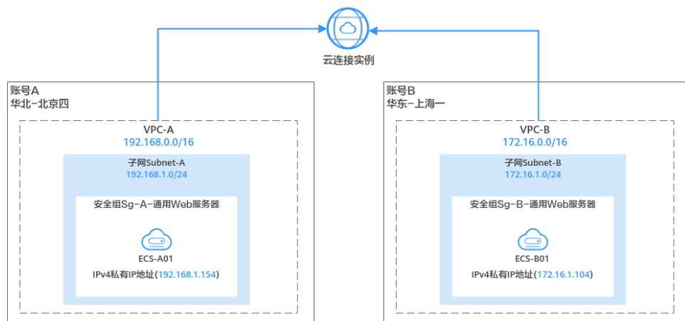
图 1-7 不同账号跨区域 VPC 互通组网规划
