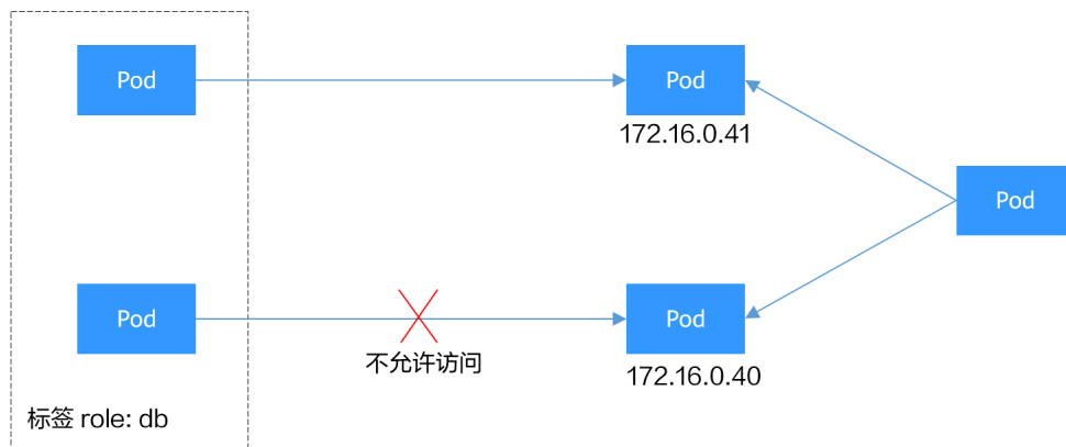
图 7-13 ipBlock
