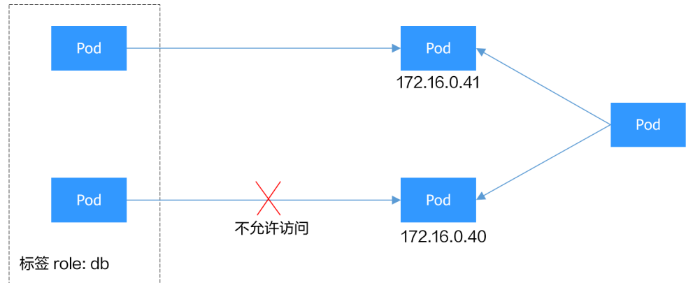
图 7-13 ipBlock
