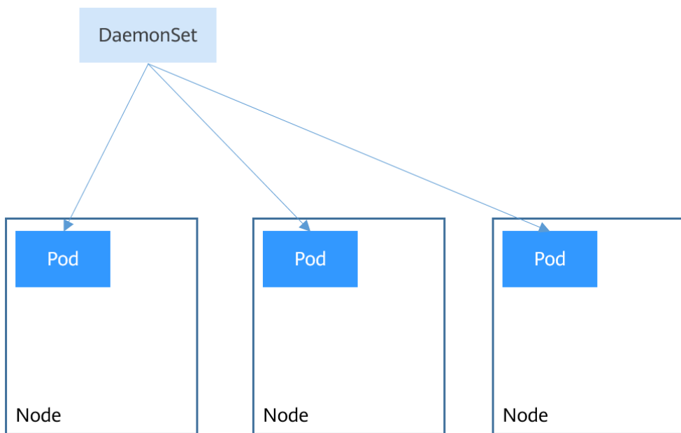
图 5-5 DaemonSet
