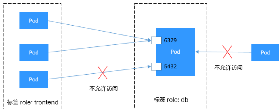
图 7-11 podSelector
