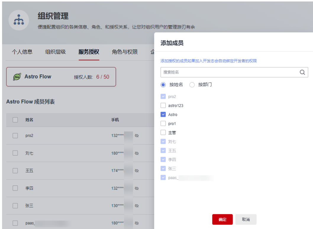
图 2-7 服务授权
