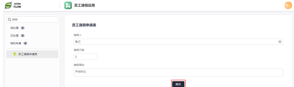
图 1-6 表单提交
