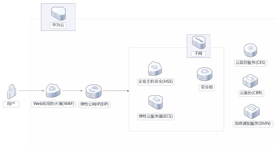
图 1-1 方案架构图
