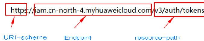
图 4-1 URI 示意图
