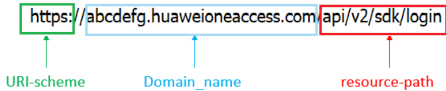
图 3-2 URI 示意图
