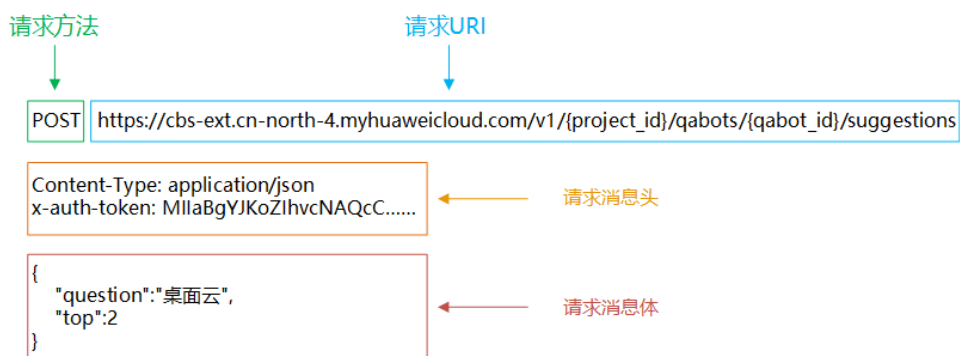
图 3-1 请求示例图
