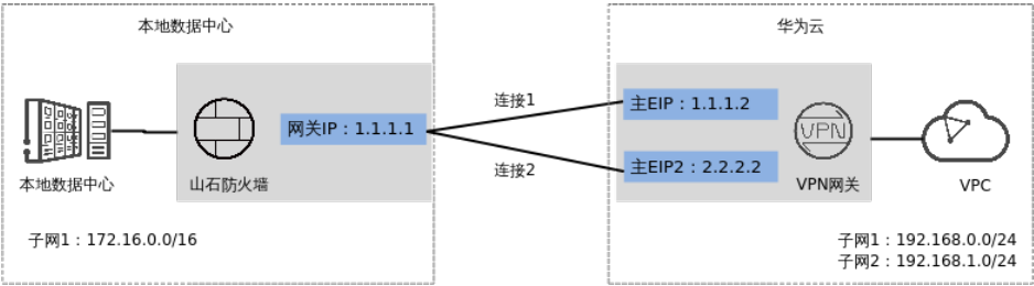
图 1-33 典型组网
