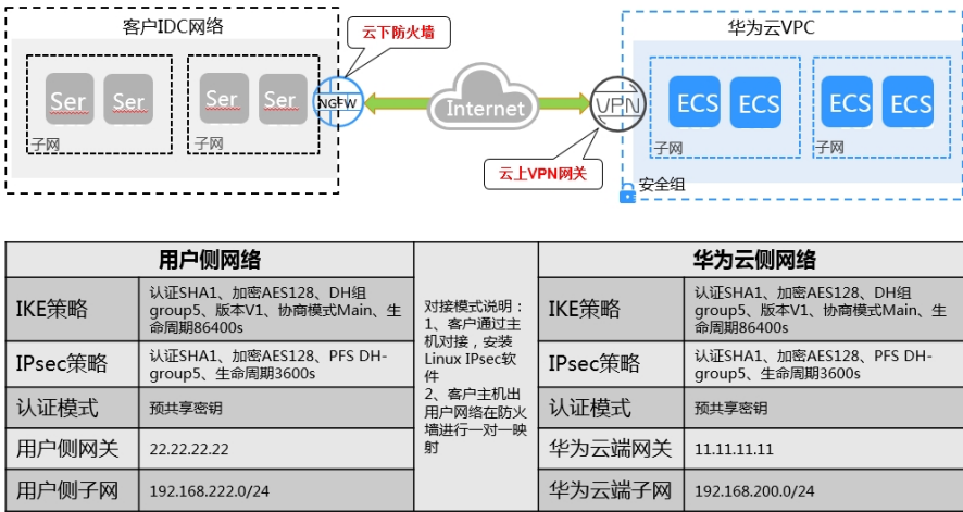
图 2-49 拓扑连接及策略协商配置信息
