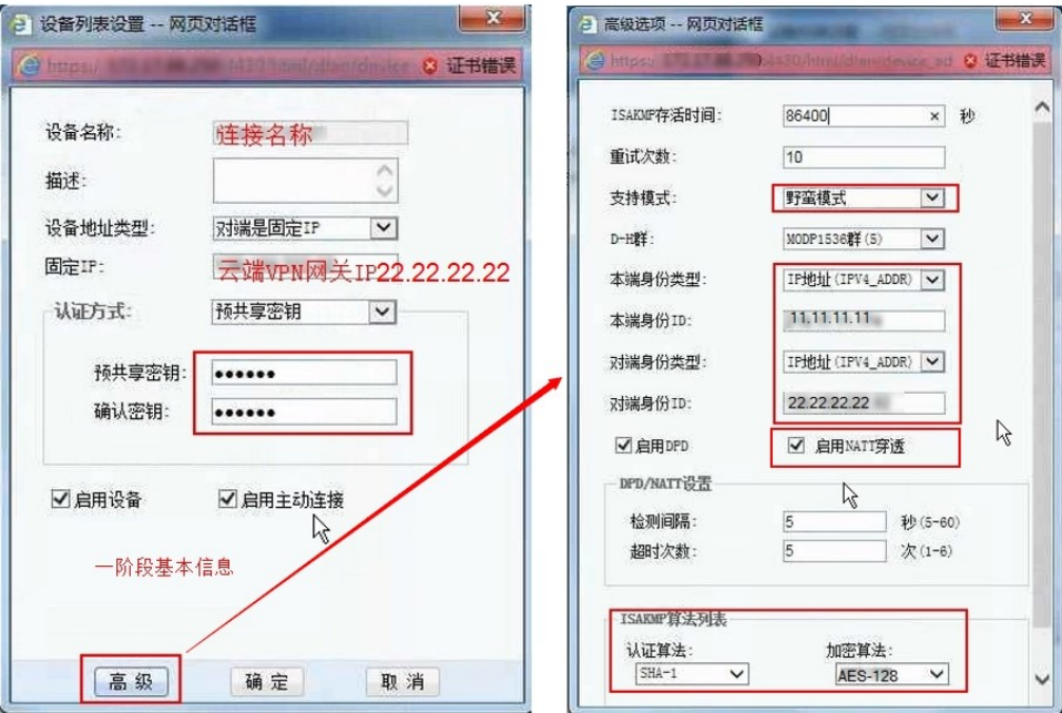
图 2-18 参数配置
