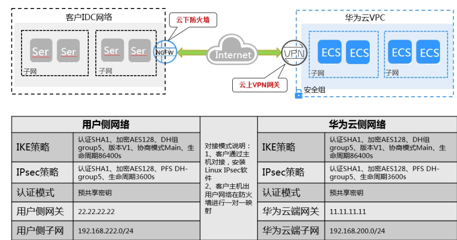
图 2-50 拓扑连接及策略协商配置信息
