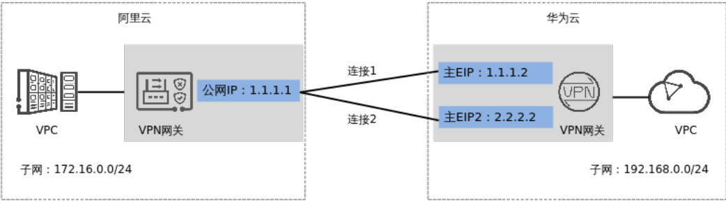
图 1-19 典型组网
