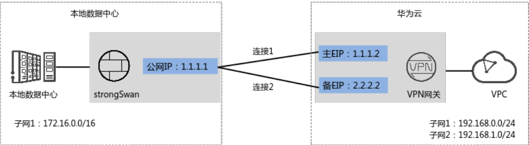
图 1-58 典型组网
