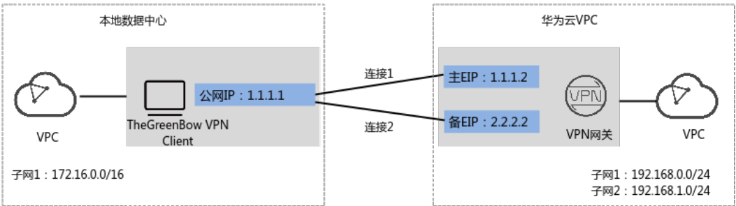
图 1-56 典型组网
