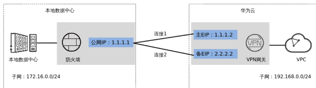
图 1-22 典型组网
