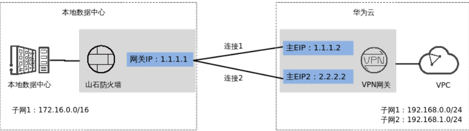
图 1-43 典型组网
