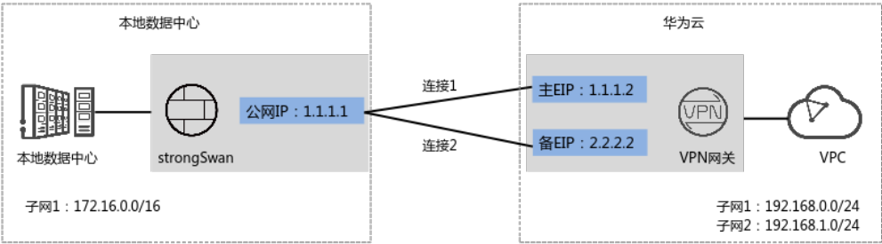
图 1-57 典型组网
