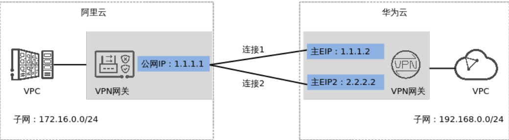
图 1-17 典型组网
