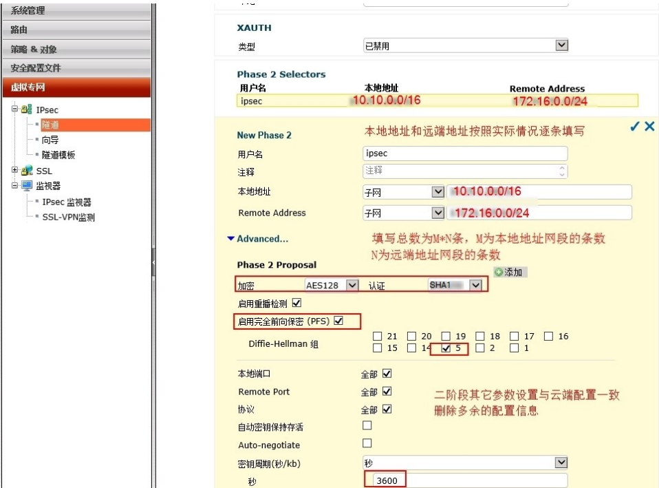
图 2-6 配置 IPsec 二阶段
