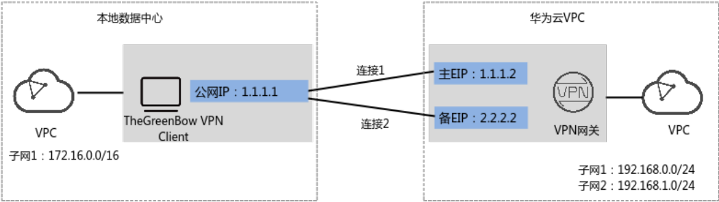
图 1-55 典型组网
