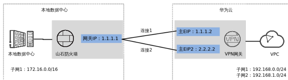
图 1-23 典型组网
