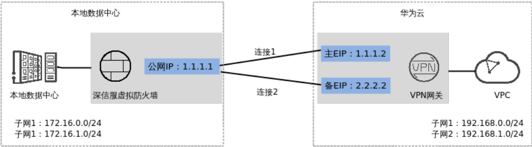
图 1-54 典型组网
