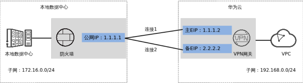
图 1-21 典型组网
