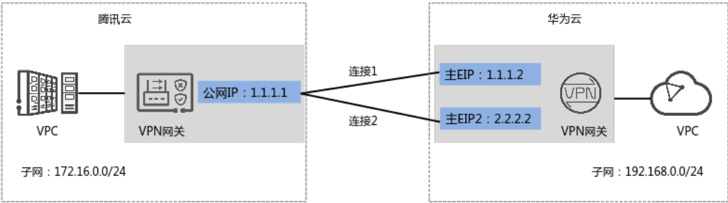
图 1-20 典型组网
