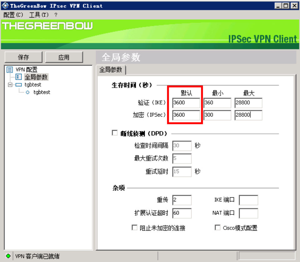
图 2-30 全局参数配置 2
