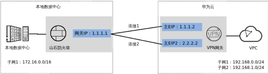
图 1-33 典型组网
