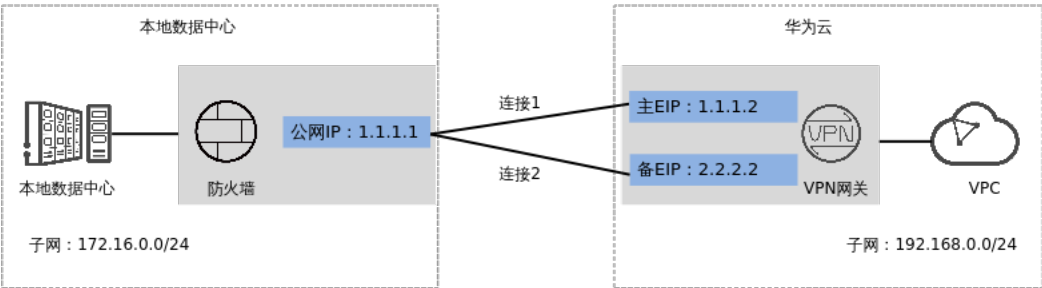
图 1-21 典型组网
