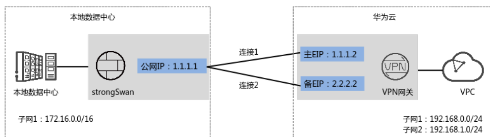
图 1-57 典型组网
